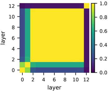
(a) raw CKA
