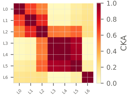
Pythia-70M: Raw CKA
