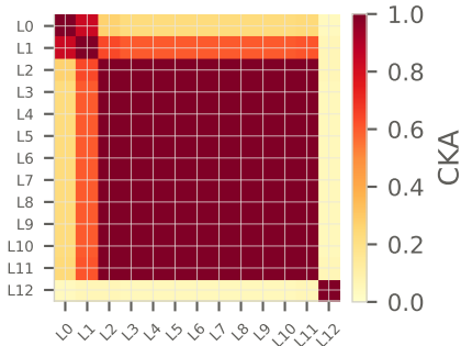
GPT-2: Raw CKA
