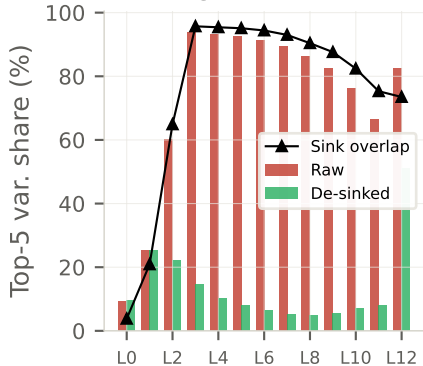
(b) Rogue dims: GPT-2
