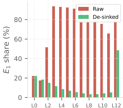
(a) E_1 : GPT-2
