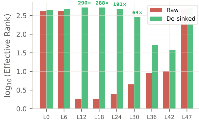
GPT-2-XL (1.5B)
