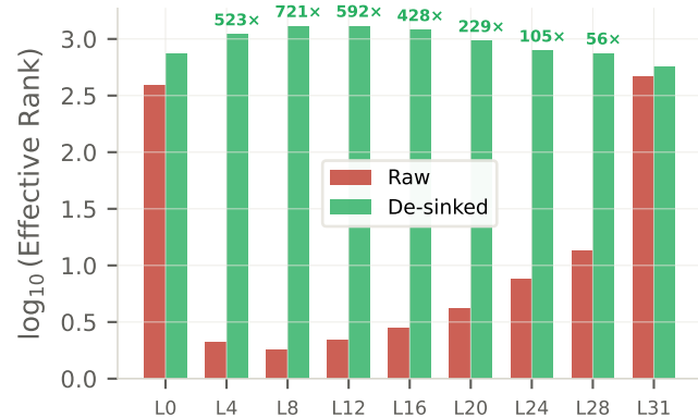
Pythia-6.9B
