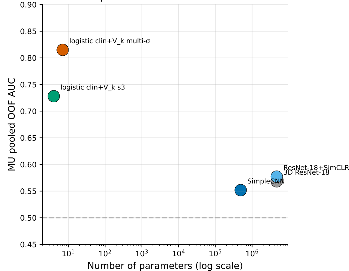
B. Parameter count vs AUC More parameters HURT at MU n=130
