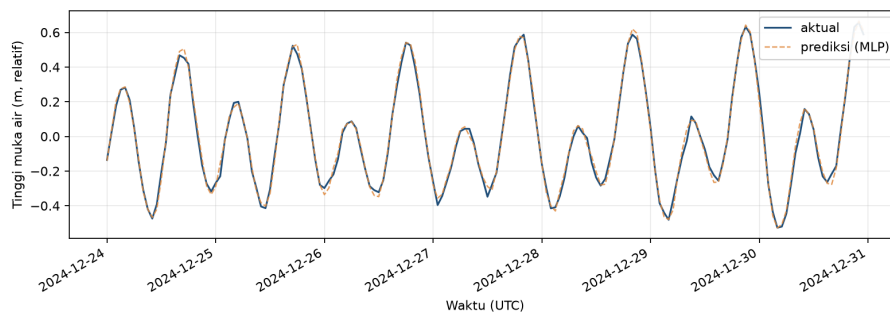
Gambar 10: Gambar 8.2 - Prediksi vs aktual 7 hari, Cilacap
