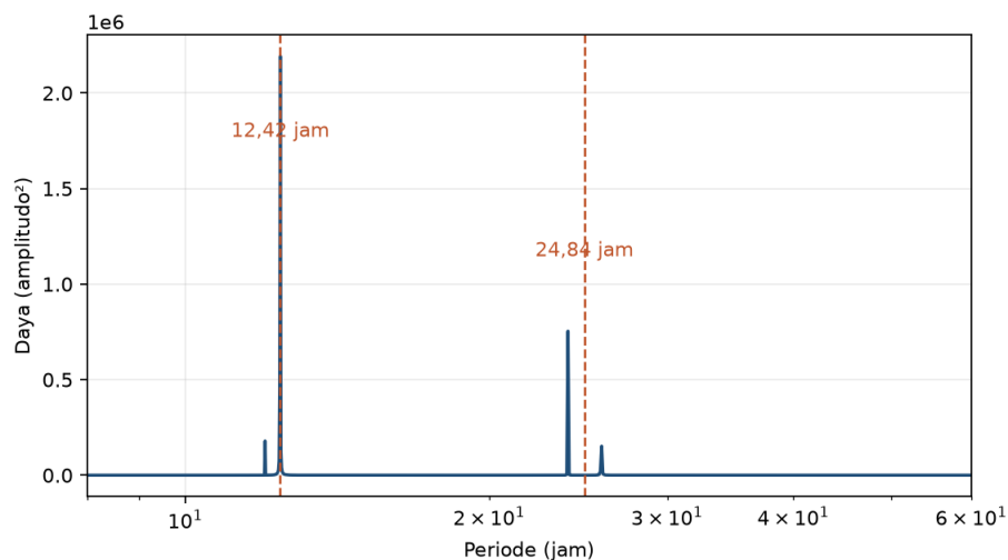
Gambar 9: Gambar 8.1 - Spektrum frekuensi muka air
