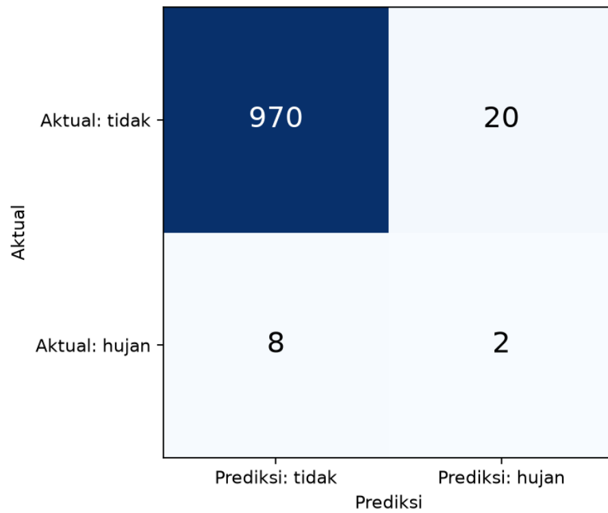
Gambar 4: Gambar 3.2 - Confusion matrix data tidak seimbang
