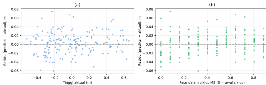
Gambar 11: Gambar 8.3 - Residu per amplitudo dan fase M2
