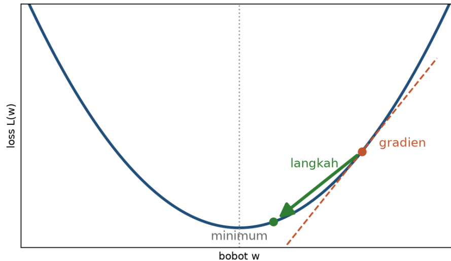
Gambar 7: Gambar 4.1 - Gradien sebagai kemiringan loss
