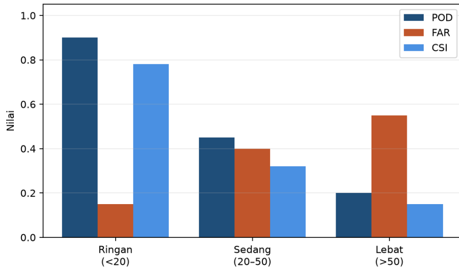
Gambar 17: Gambar 9.2 - Verifikasi per kategori intensitas
