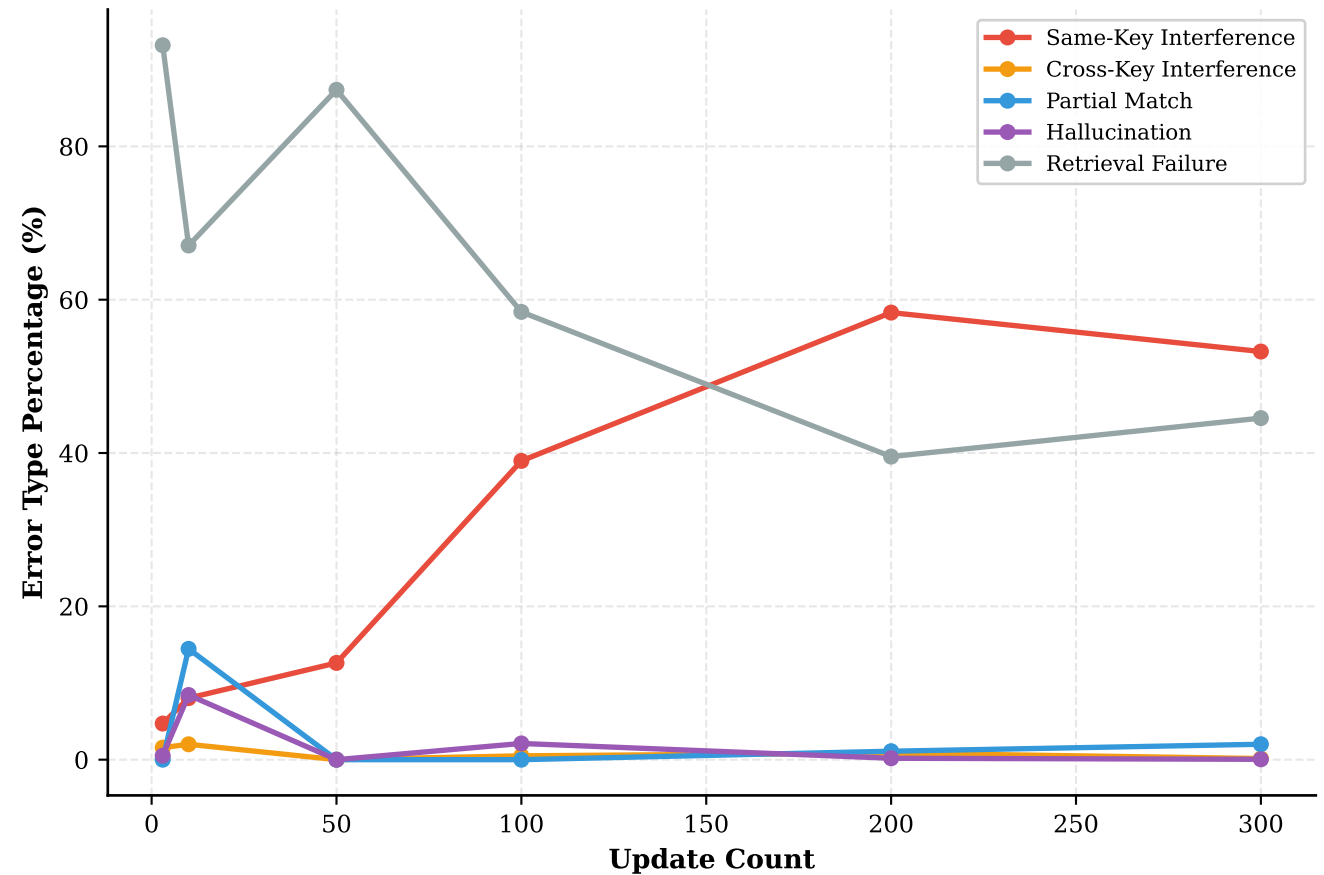
Error Type Trajectories
