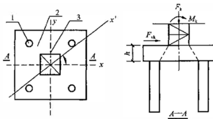
图 3.2.4 塔式起重机方形承台桩基础
