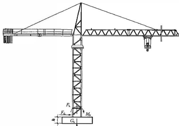
图 3.2.3 塔式起重机板式基础计算简图
