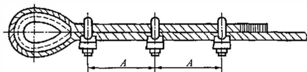
图 6.2.4 钢丝绳夹压板布置图
