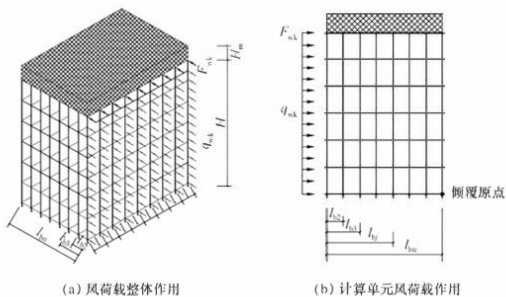
图 6.2.15 风荷载作用示意
