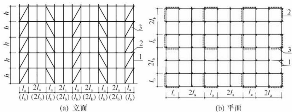
图 8.3.5-1 竖向斜撑杆布置示意（一） 1—立杆；2—水平杆；3—斜撑杆
