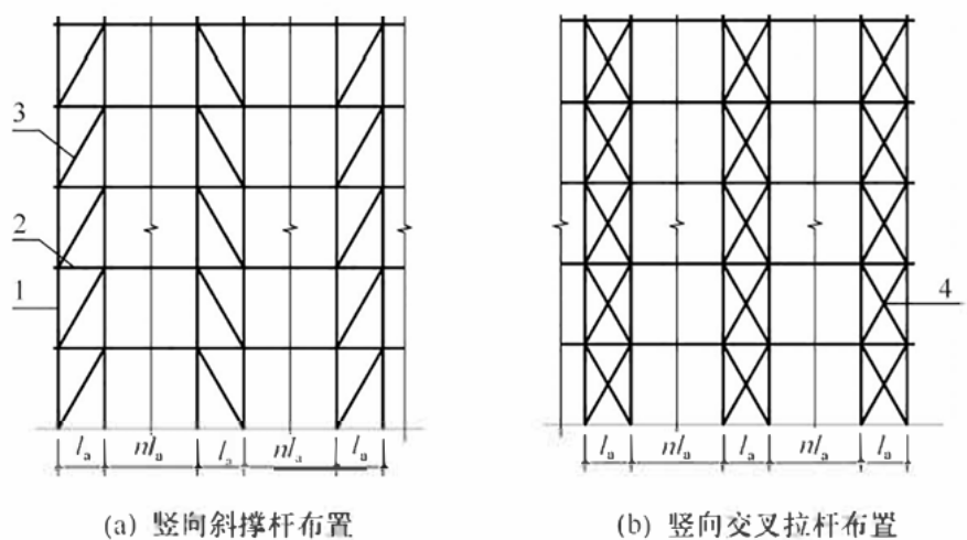
图 8.2.4 作业脚手架竖向斜撑杆布置示意 1—立杆；2—水平杆；3—斜撑杆；4—交叉拉杆
