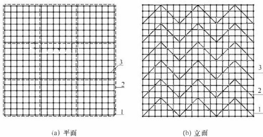
图 8.3.5-2 竖向斜撑杆布置示意 (二)
