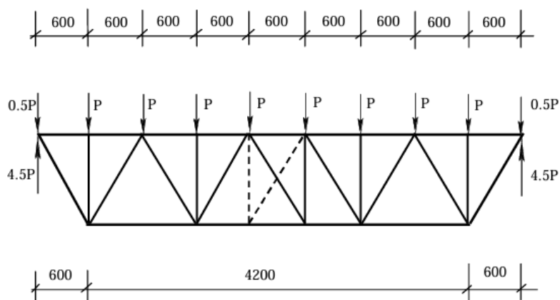
图 5.2.2—3 可调桁架跨长计算简图示意
