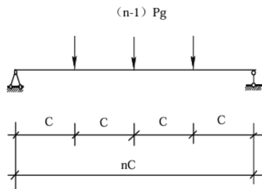
图 5.2.2—4 桁架节点集中荷载布置图（偶数节间）
