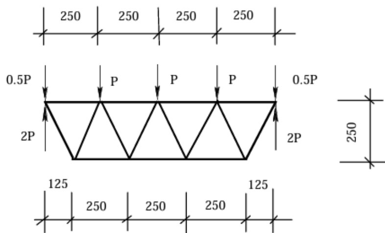
图 5.2.2—1 轻型桁架计算简图示意
