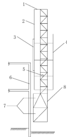
图 5.3.1 爬模组成
