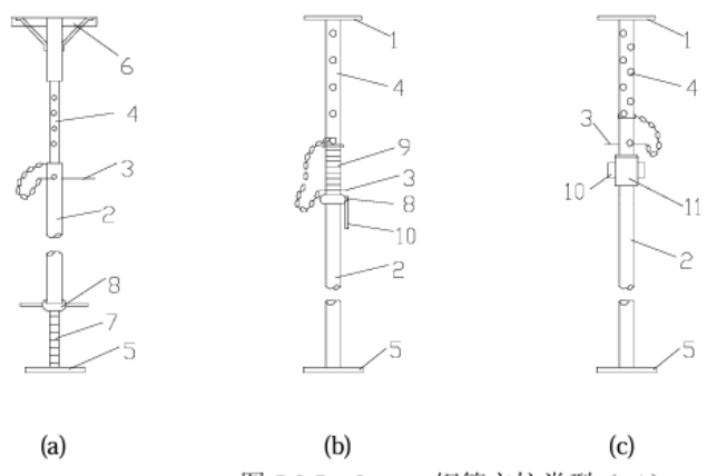
图 5.2.5—2 钢管立柱类型（二）
