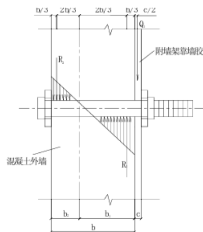
图 5.3.5—2 螺栓孔混凝土承压计算
