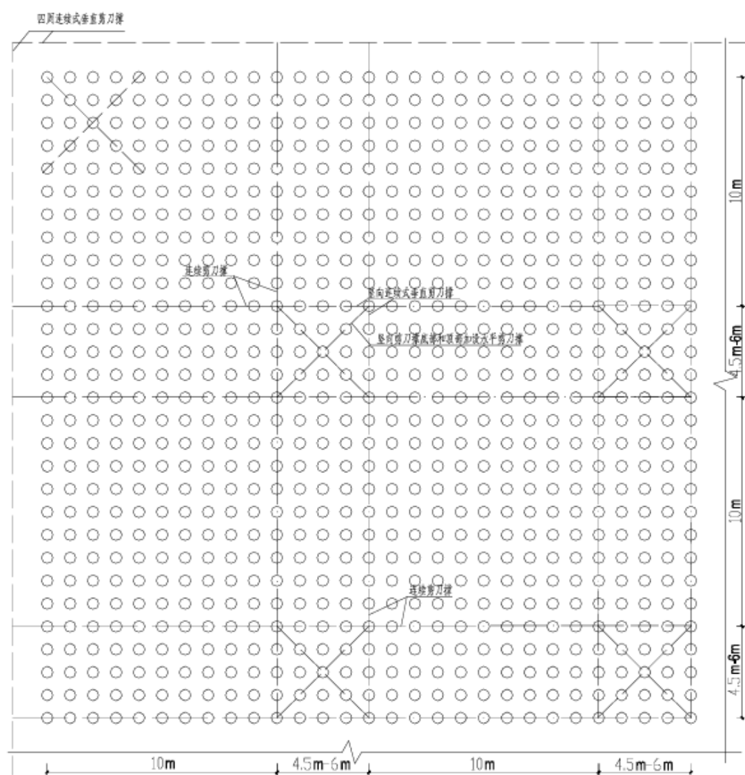
图 6.2.4—3 剪刀撑布置图三
