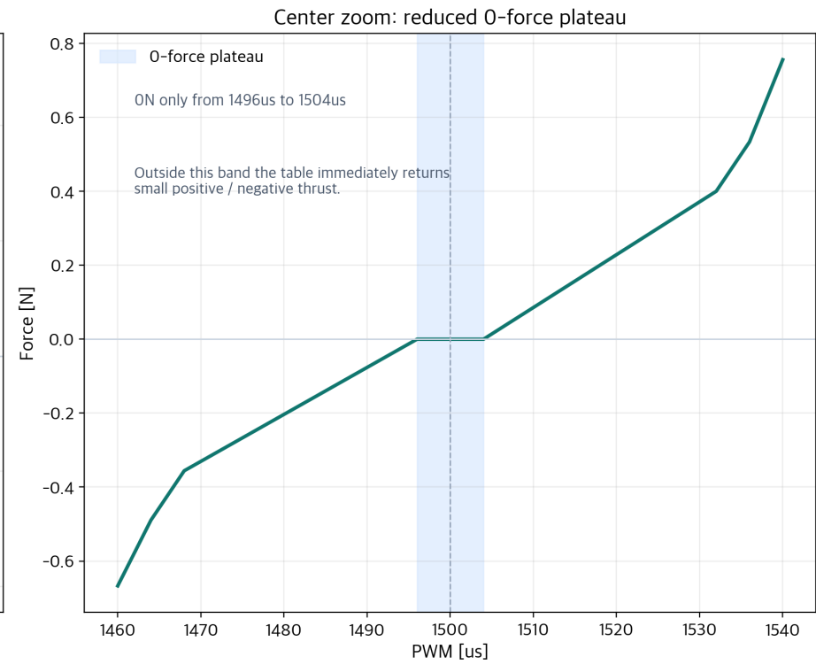
Figure 3: 16V T200 performance reference graph. 좌측은 전체 force curve, 우측은 1500 us 주변 0-force plateau 축소 구간을 확대해 보여준다.
