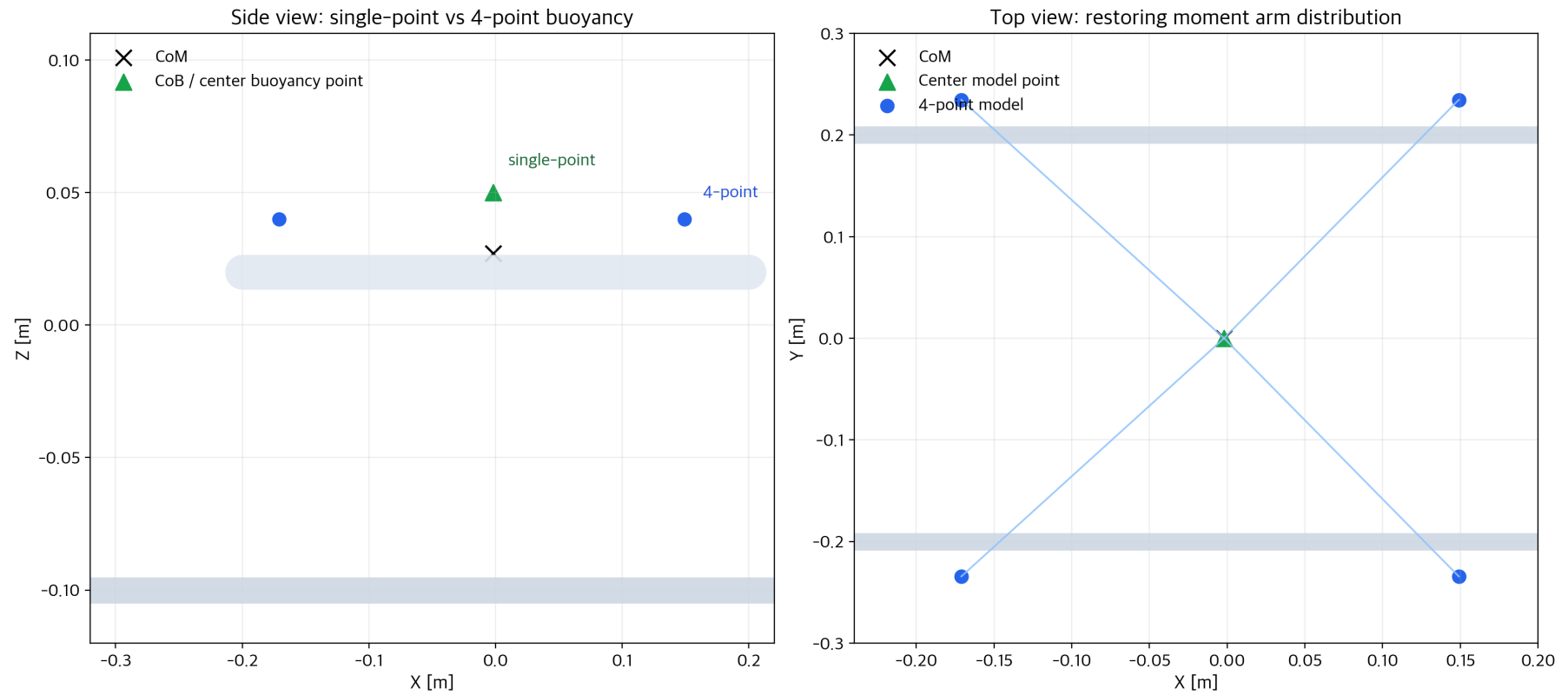
Figure 4: single-point center와 current 4-point buoyancy layout 비교. 같은 총 부력을 어디에 어떻게 분포시키는지의 차이를 시각적으로 보여준다.
