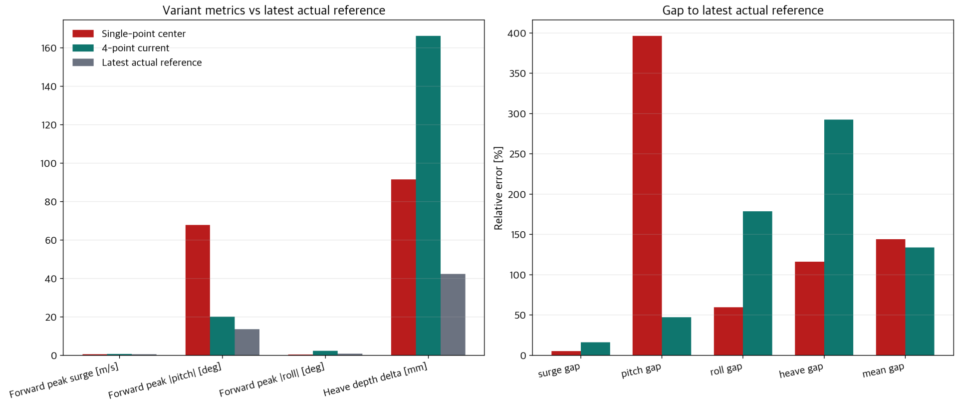
Figure 6: latest actual reference 대비 key metric과 상대 오차 비교. peak surge, peak pitch / roll, heave depth delta, mean gap을 요약했다.
