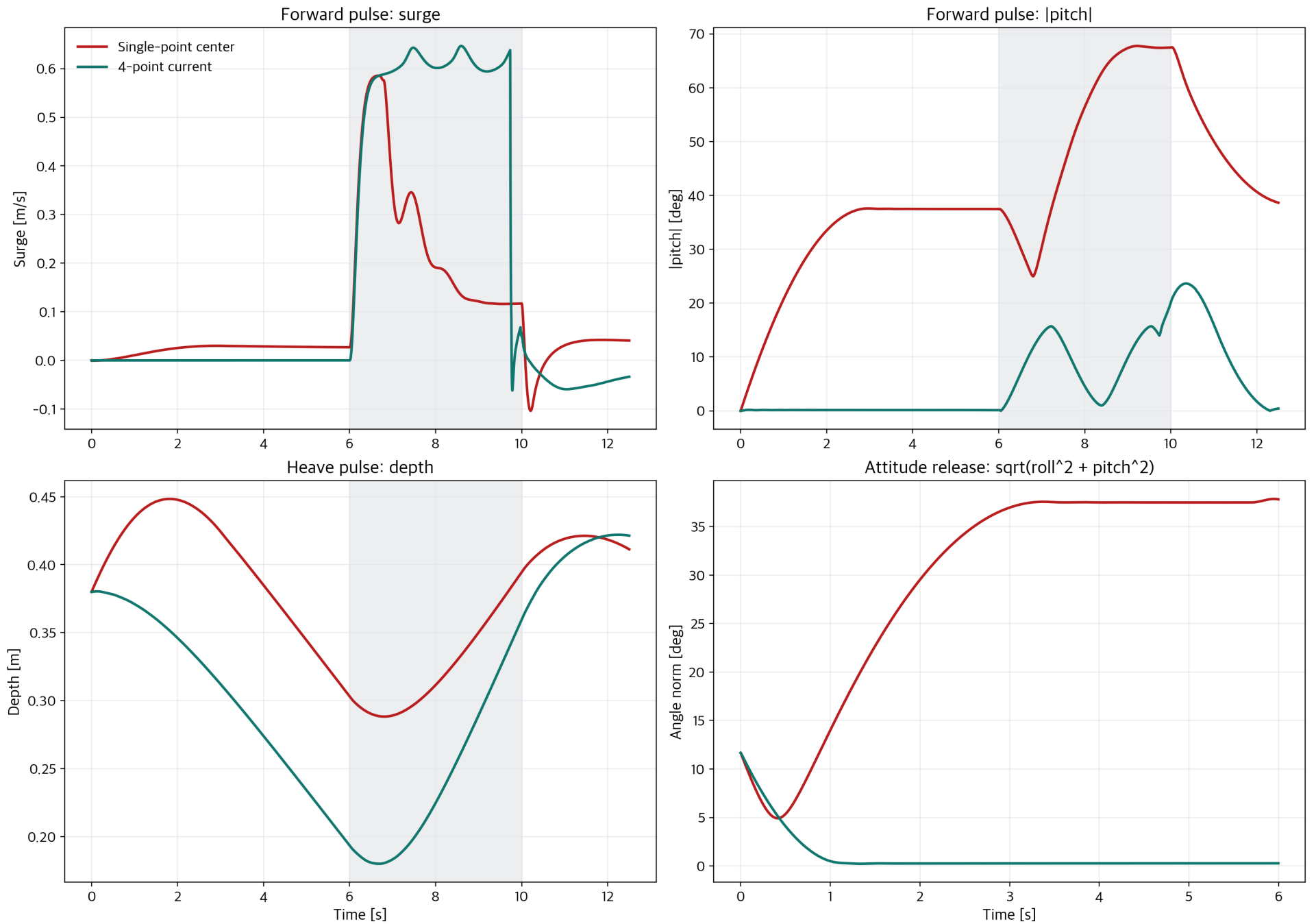
Figure 5: 같은 current scene / thrust model / scripted harness에서 buoyancy 구성만 바꾼 응답 비교. 전진, pitch, heave, attitude release를 한 장에 묶었다.
