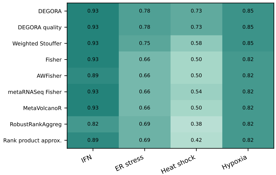
B. Recall@100
