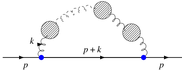
图 5-1 夸克自能修正图中的链式泡沫图
