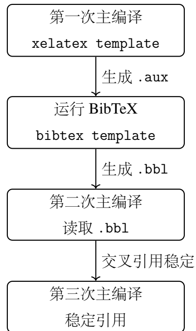
图 B-1 BibTeX 参考文献编译流程示意图
