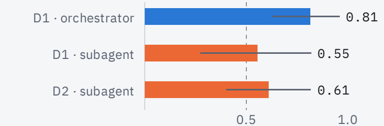
트레이스 수준 AUROC (max 요약, 실패 25 / 성공 6 · §4.2.3)
