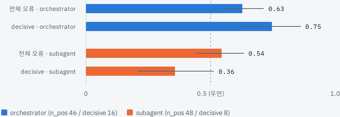
스텝 수준 AUROC (1 - p_actual, 95 % CI · §4.2.2)
