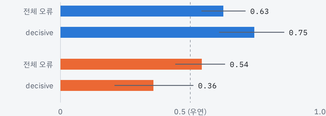
스텝 수준 AUROC (1 - p_actual, 95 % CI · §4.2.2)
