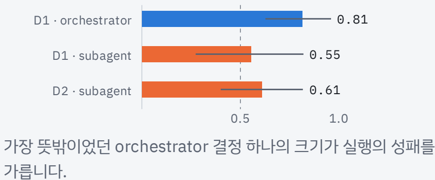
트레이스 수준 AUROC (max 요약, 실패 25 / 성공 6 · §4.2.3)
