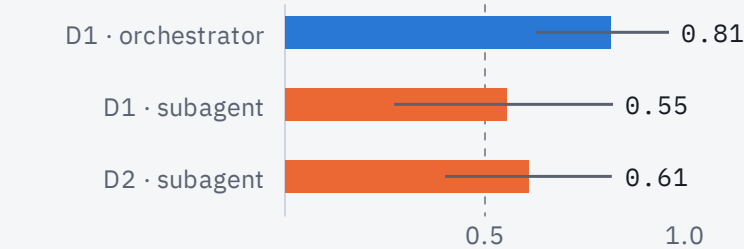
트레이스 AUROC (MAX 요약, 실패 25 / 성공 6)
