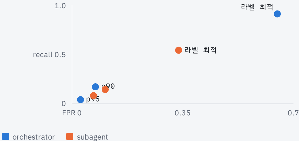
백분위 임계값 대 라벨 최적 (D1 1 - CONFIDENCE)
