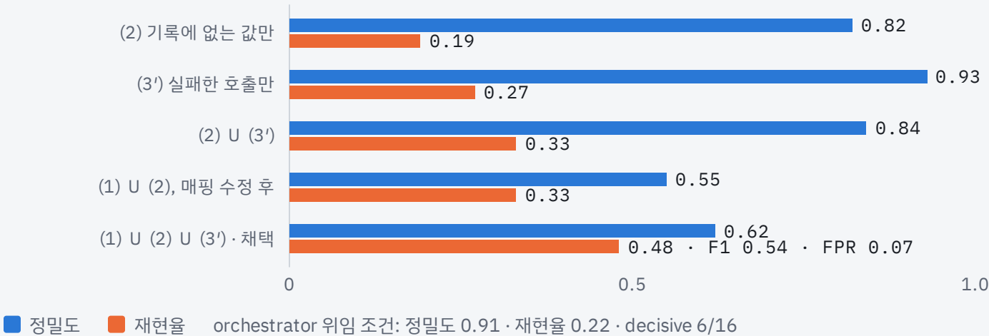
D2 구성별 정밀도와 재현율 (SUBAGENT, 양성 48 / 음성 190)
