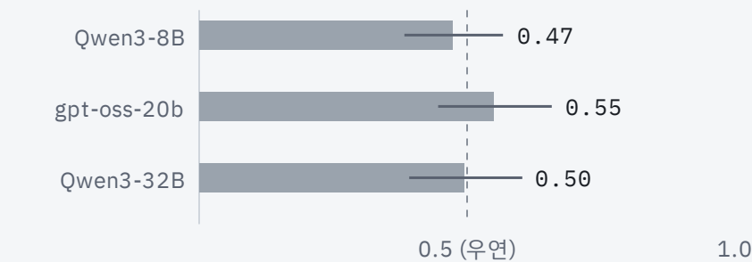
D4 · 판정기 세 종, AIRLINE SUBAGENT AUROC (95 % CI)
