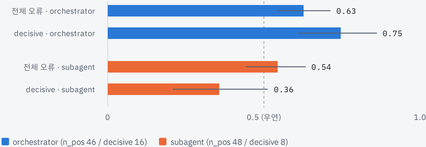
스텝 AUROC (1 - P_ACTUAL, 95 % CI)
