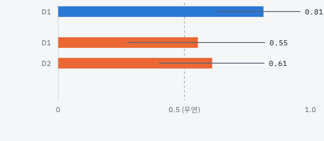
트레이스 수준 AUROC (max 요약, 실패 25 / 성공 6 · §4.2.3)
