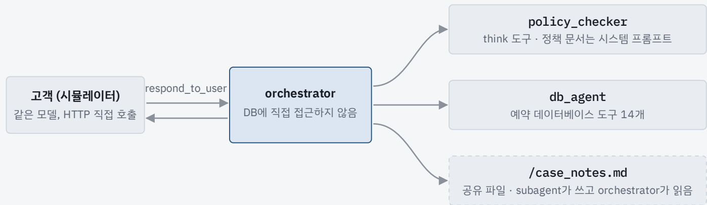
래퍼 도구 policy_checker / db_agent 호출 → subagent 그래프 실행 → 보고서가 도구 결과로 돌아옴
