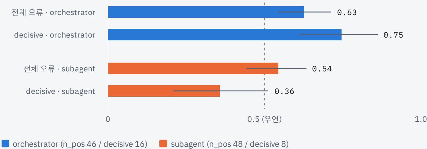
스텝 AUROC (1 - P_ACTUAL, 95 % CI)
