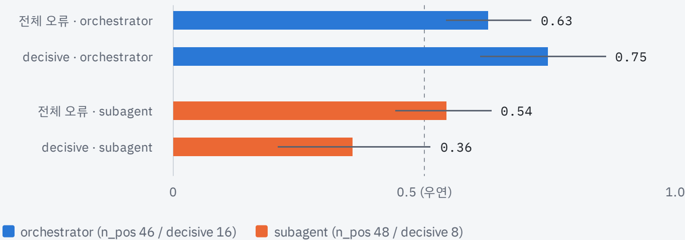
스텝 수준 AUROC (1 - p_actual, 95 % CI · §4.2.2)
