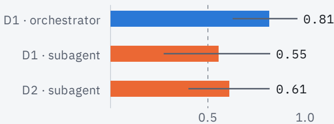
트레이스 수준 AUROC (max 요약, 실패 25 / 성공 6 · §4.2.3)
