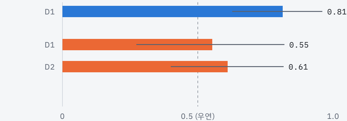
트레이스 수준 AUROC (max 요약, 실패 25 / 성공 6 · §4.2.3)
