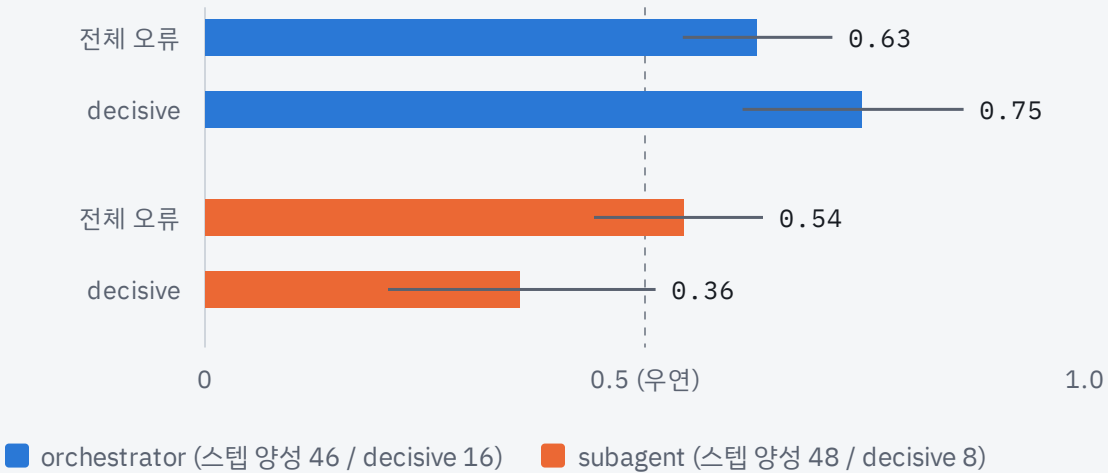
스텝 수준 AUROC (1 - p_actual, 95 % CI · §4.2.2)
