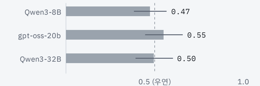
D4 판정기 세 종 비교 (airline subagent AUROC (95 % CI) · §4.2.13)
