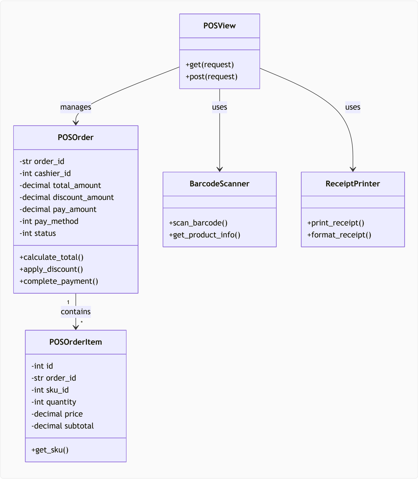
3.7.4 POS模块内部交互拓扑图
