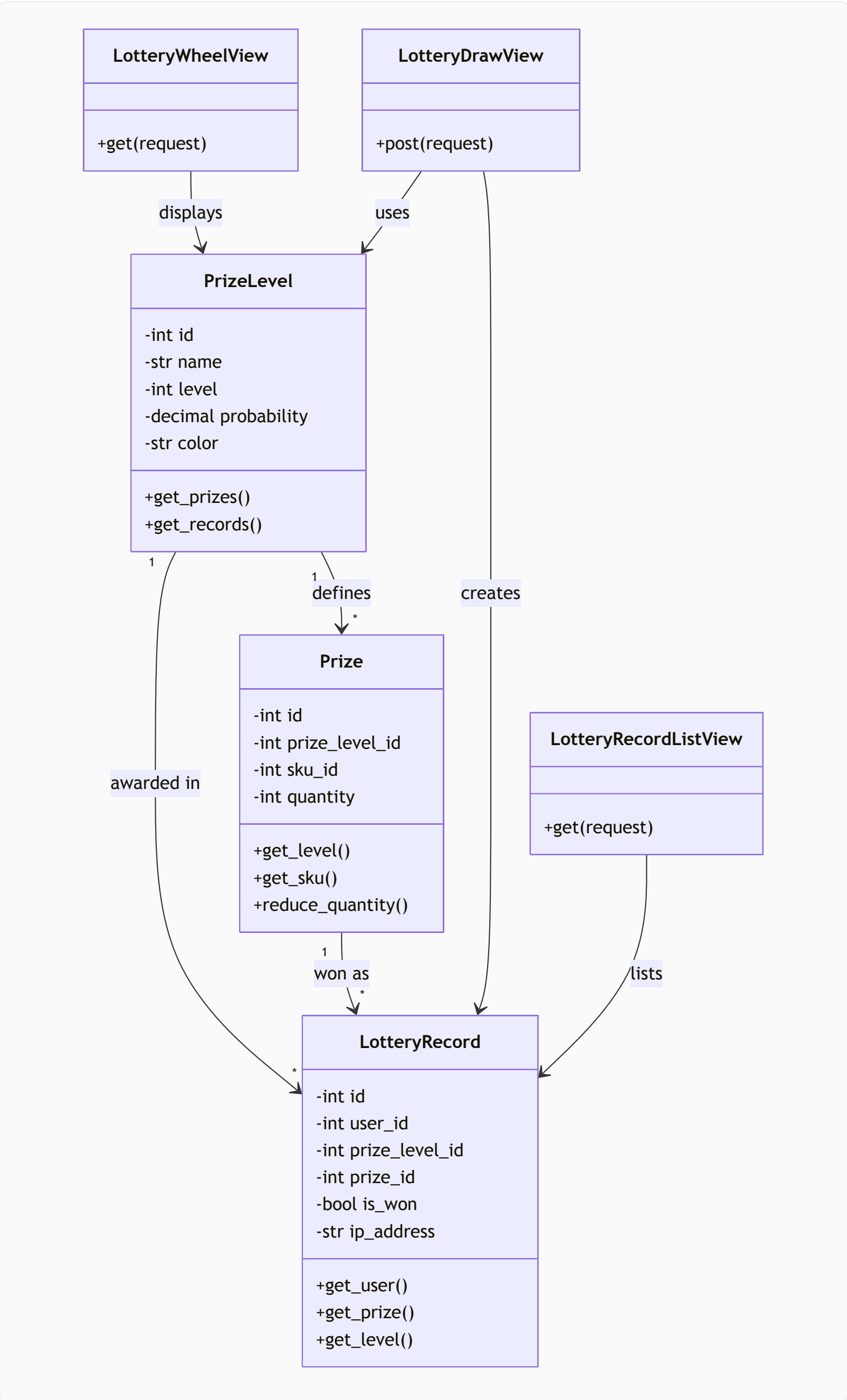
3.6.4 抽奖模块内部交互拓扑图
