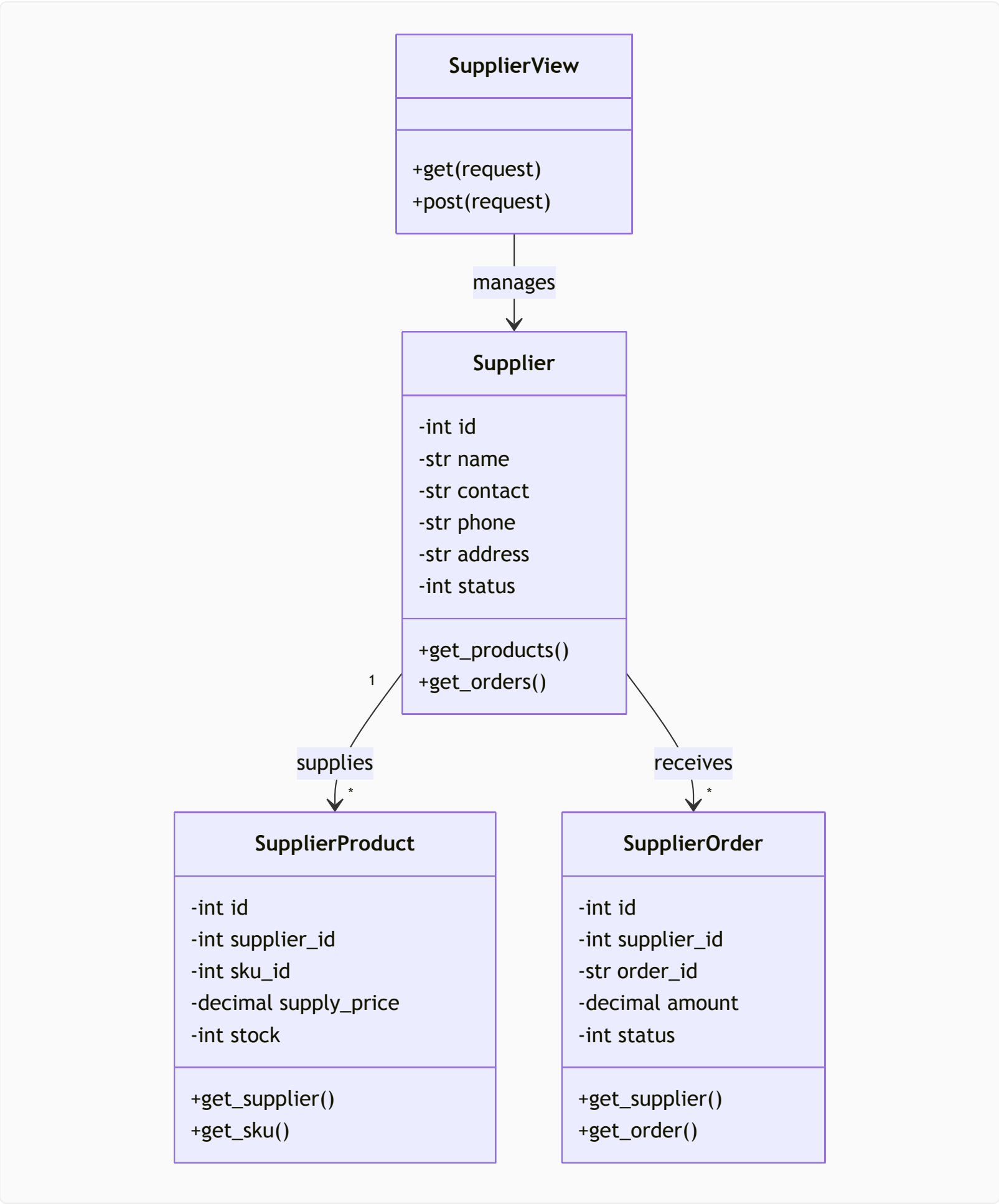
3.8.4 供应商模块内部交互拓扑图
