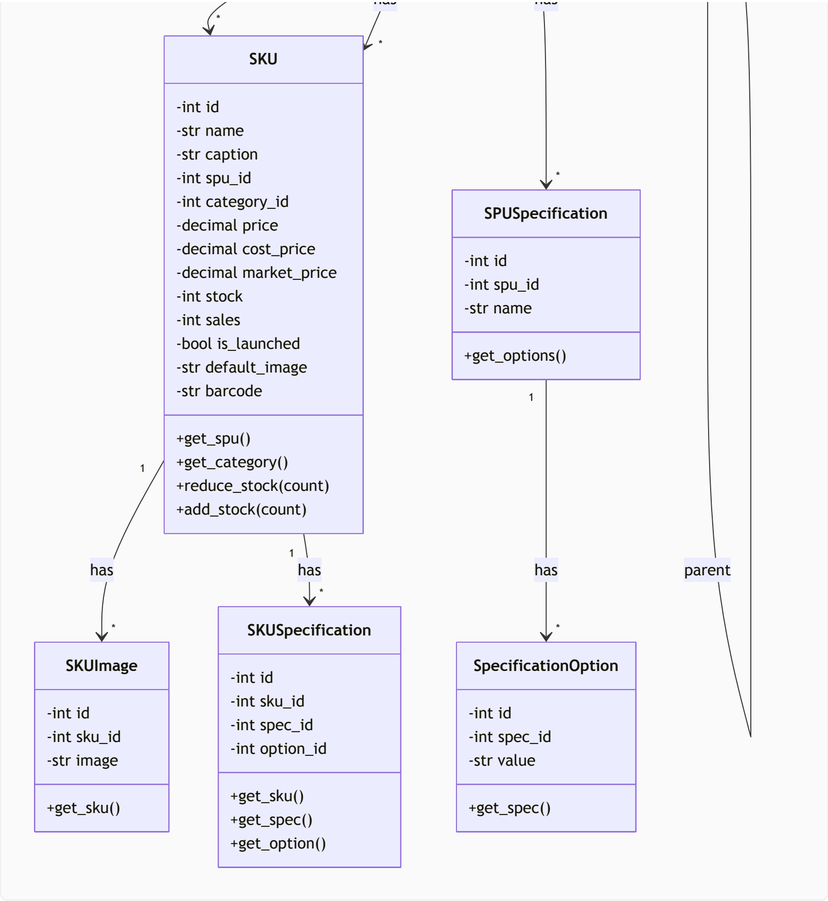
3.2.4 商品模块内部交互拓扑图
