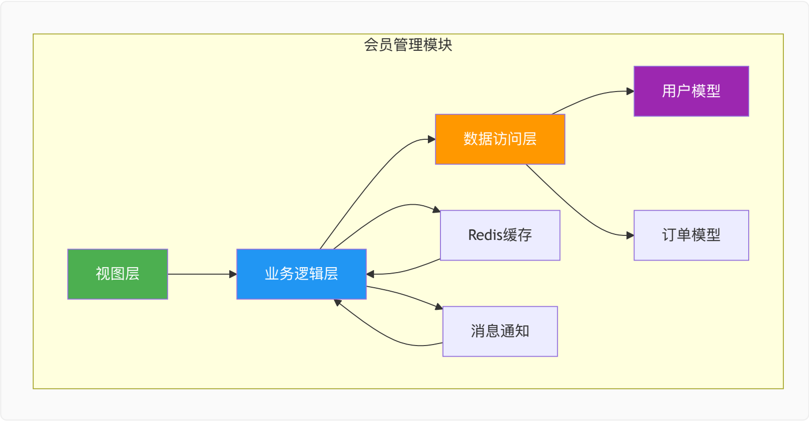
3.11.5 会员管理模块业务流程图
