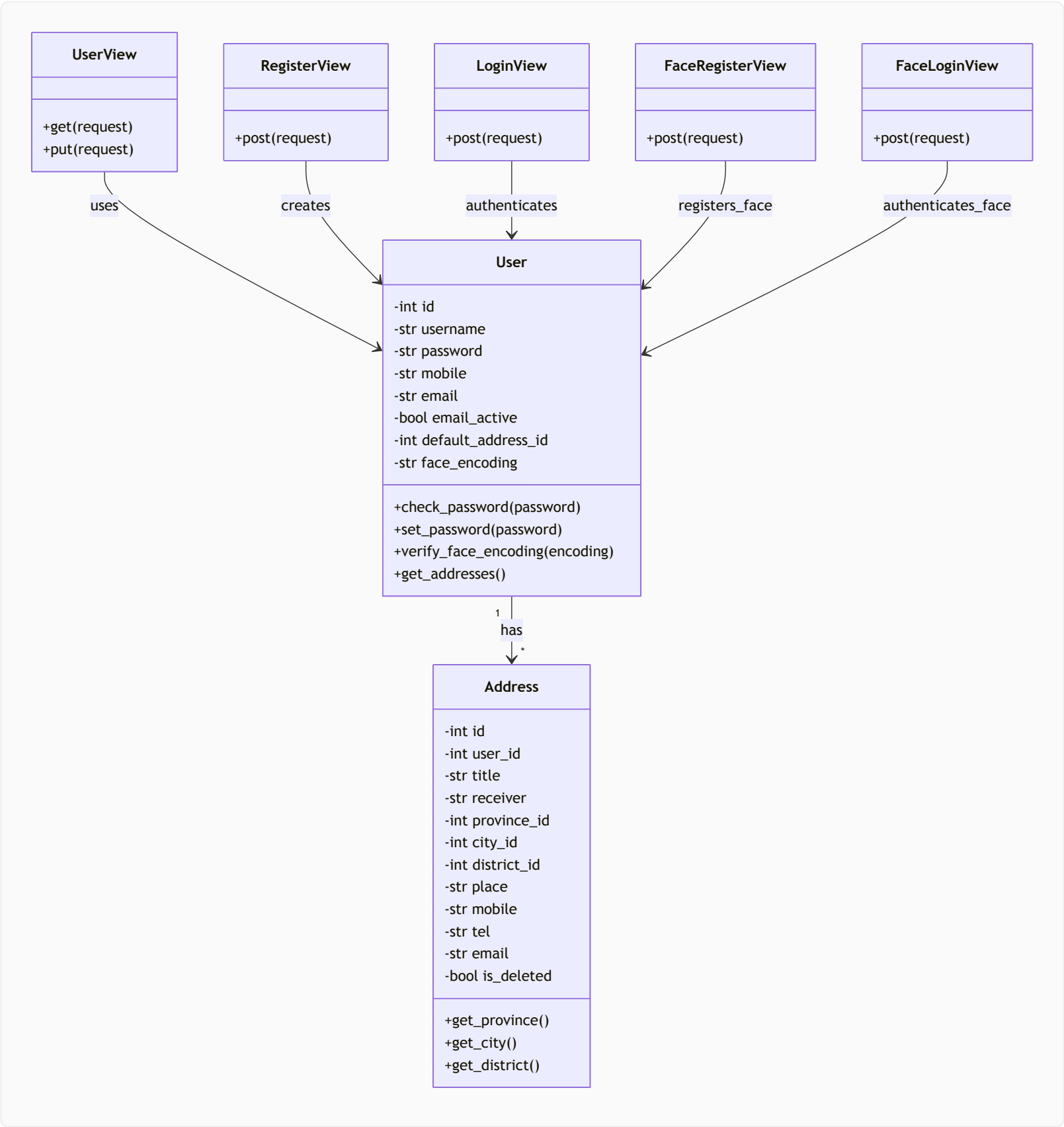
3.1.4 用户模块内部交互拓扑图
