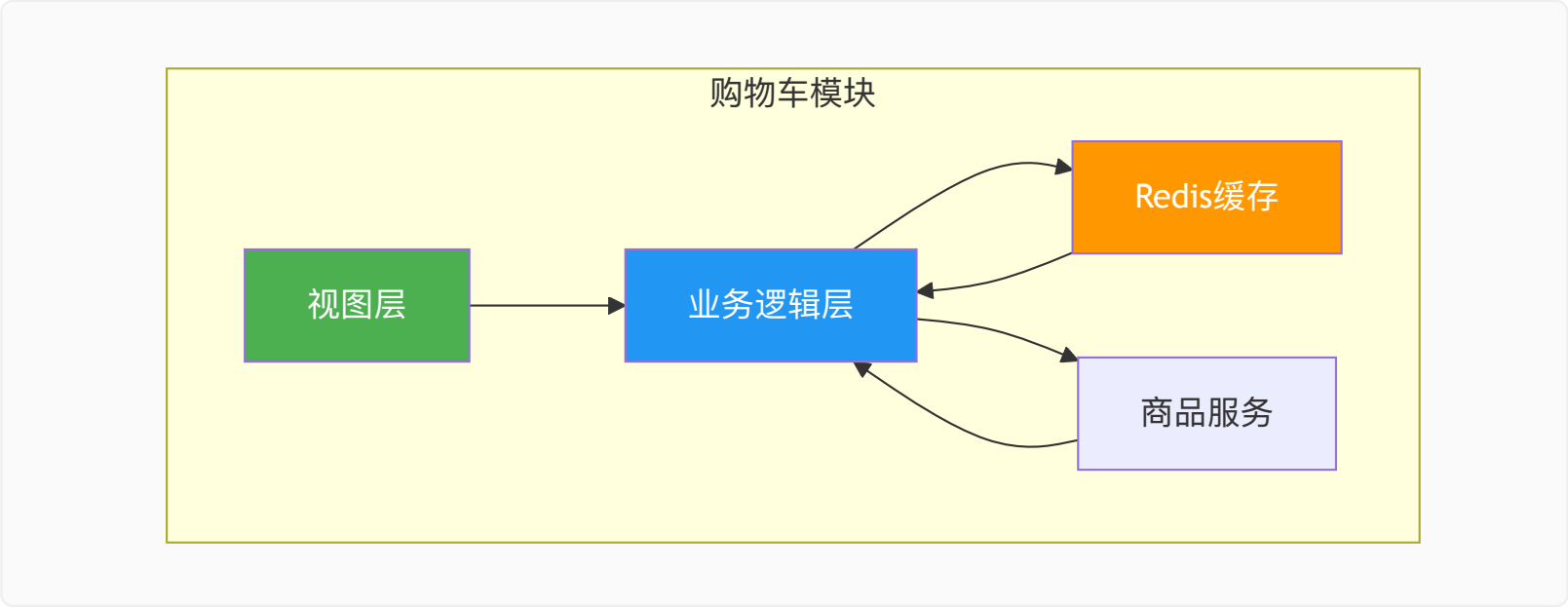
3.5.4 购物车模块内部交互拓扑图
