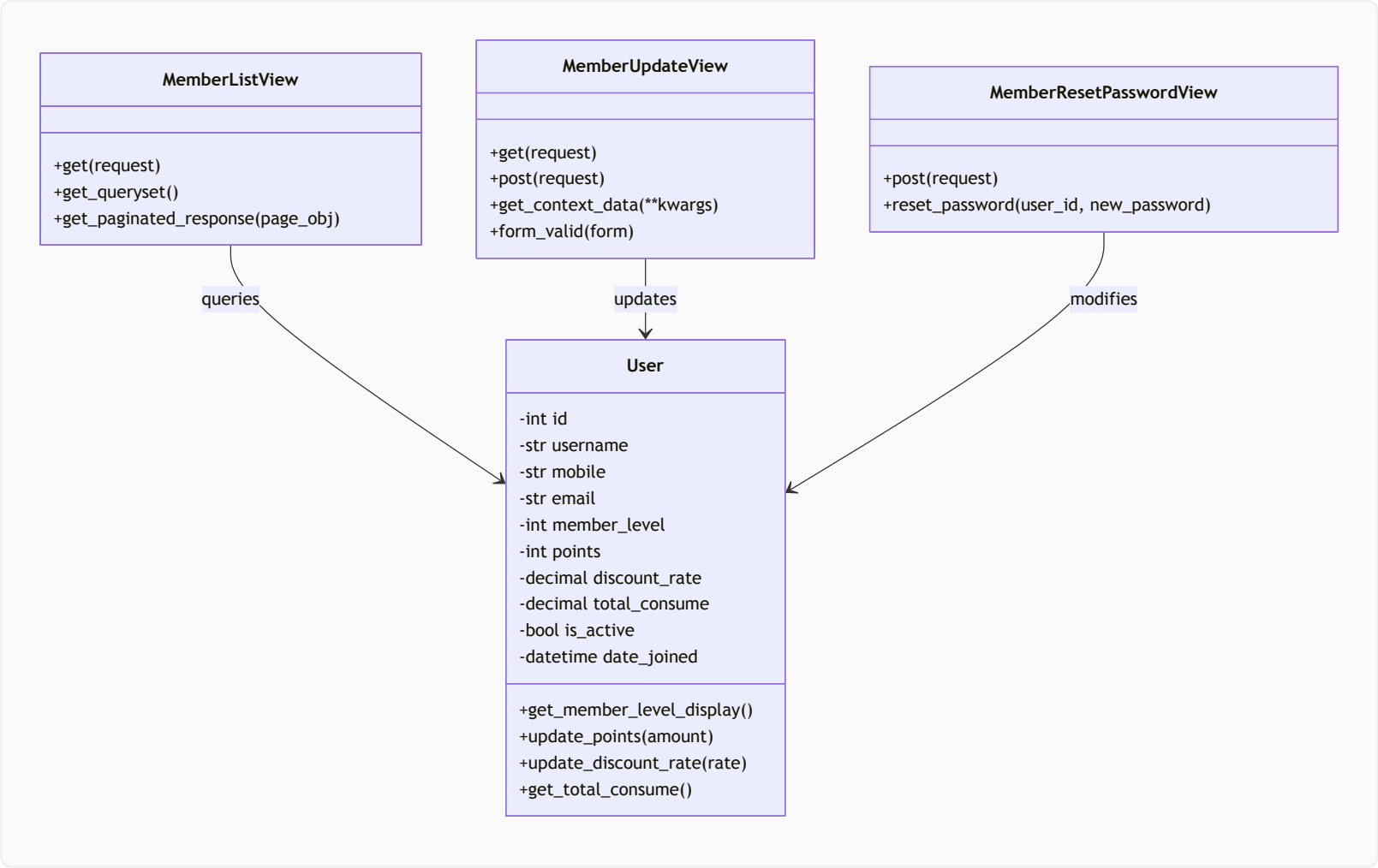
3.11.4 会员管理模块内部交互拓扑图
