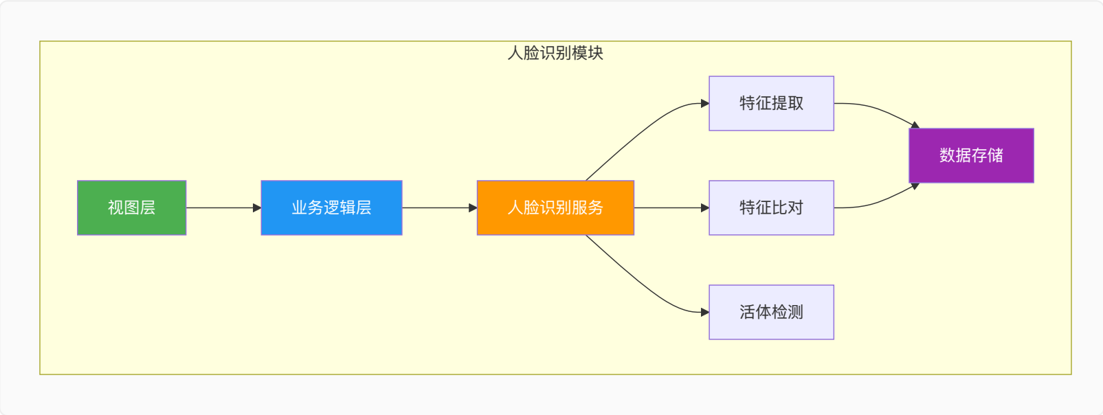
3.10.4 人脸识别模块内部交互拓扑图
