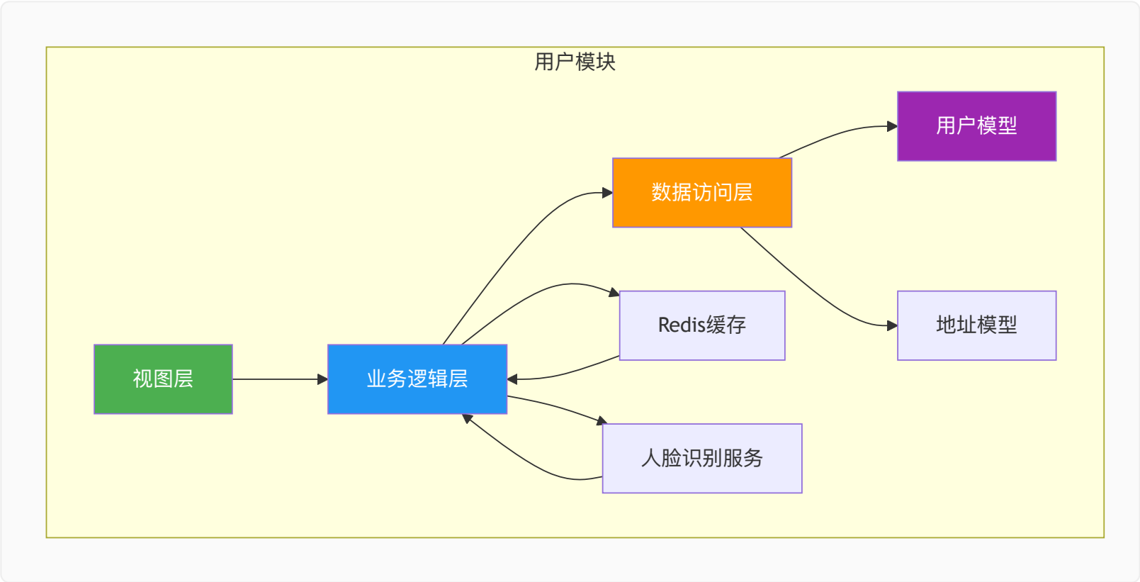
3.1.4 用户模块内部交互拓扑图
