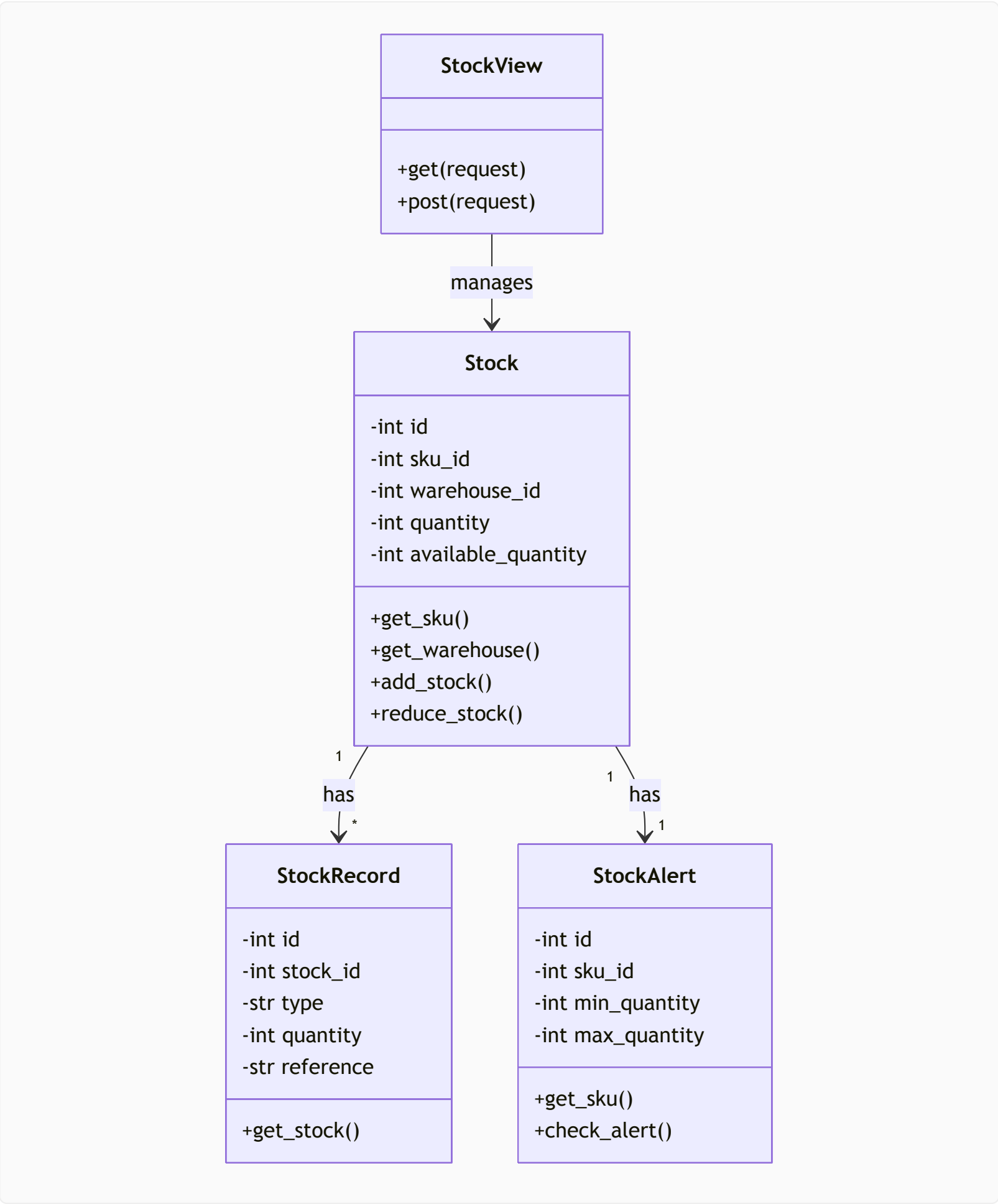
3.9.4 库存模块内部交互拓扑图
