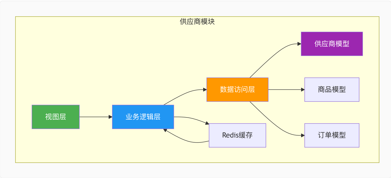
3.8.4 供应商模块内部交互拓扑图
