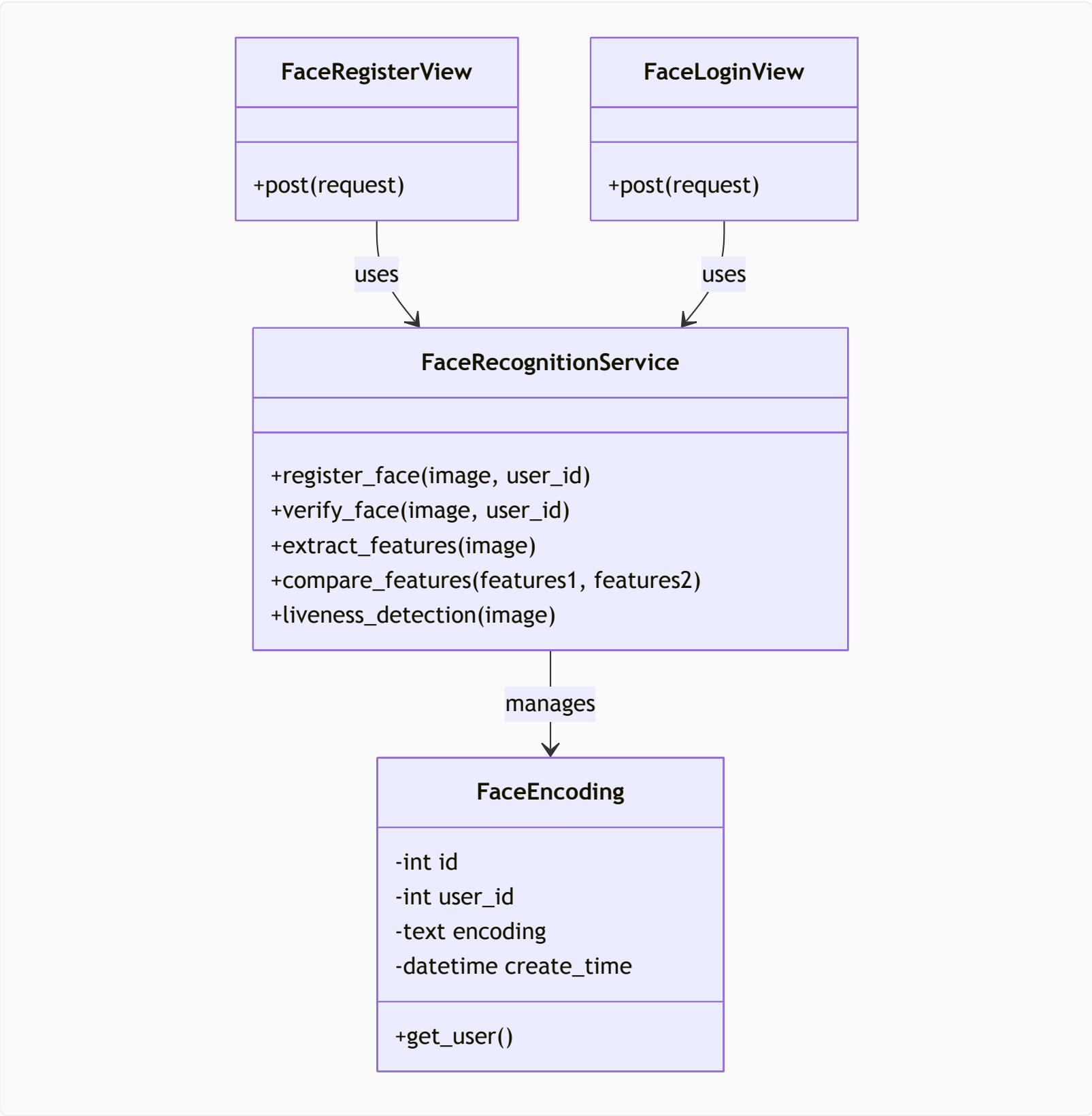
3.10.4 人脸识别模块内部交互拓扑图
