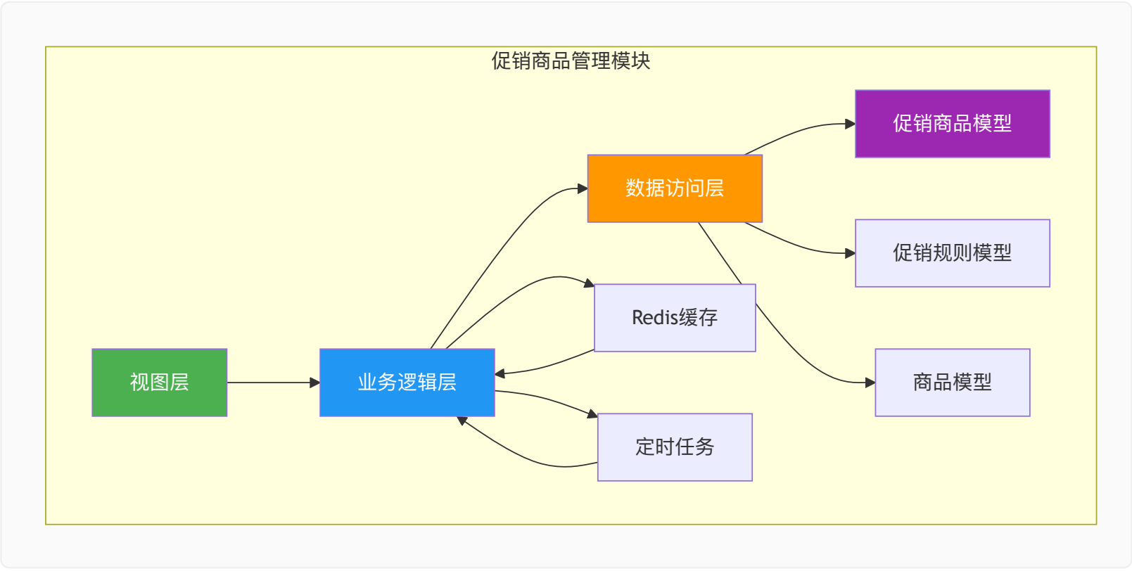
3.12.5 促销商品管理流程图
