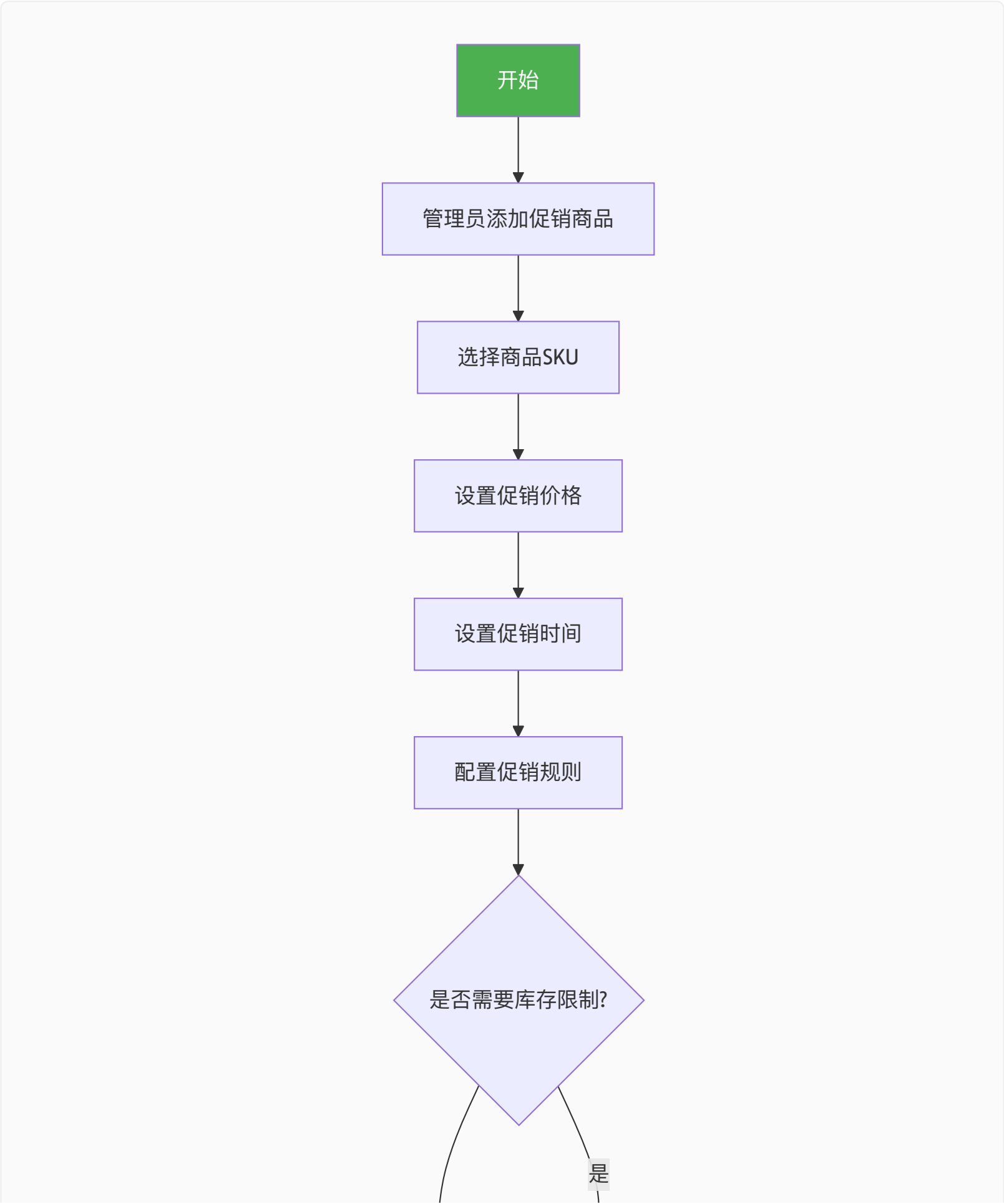
3.12.5 促销商品管理流程图
