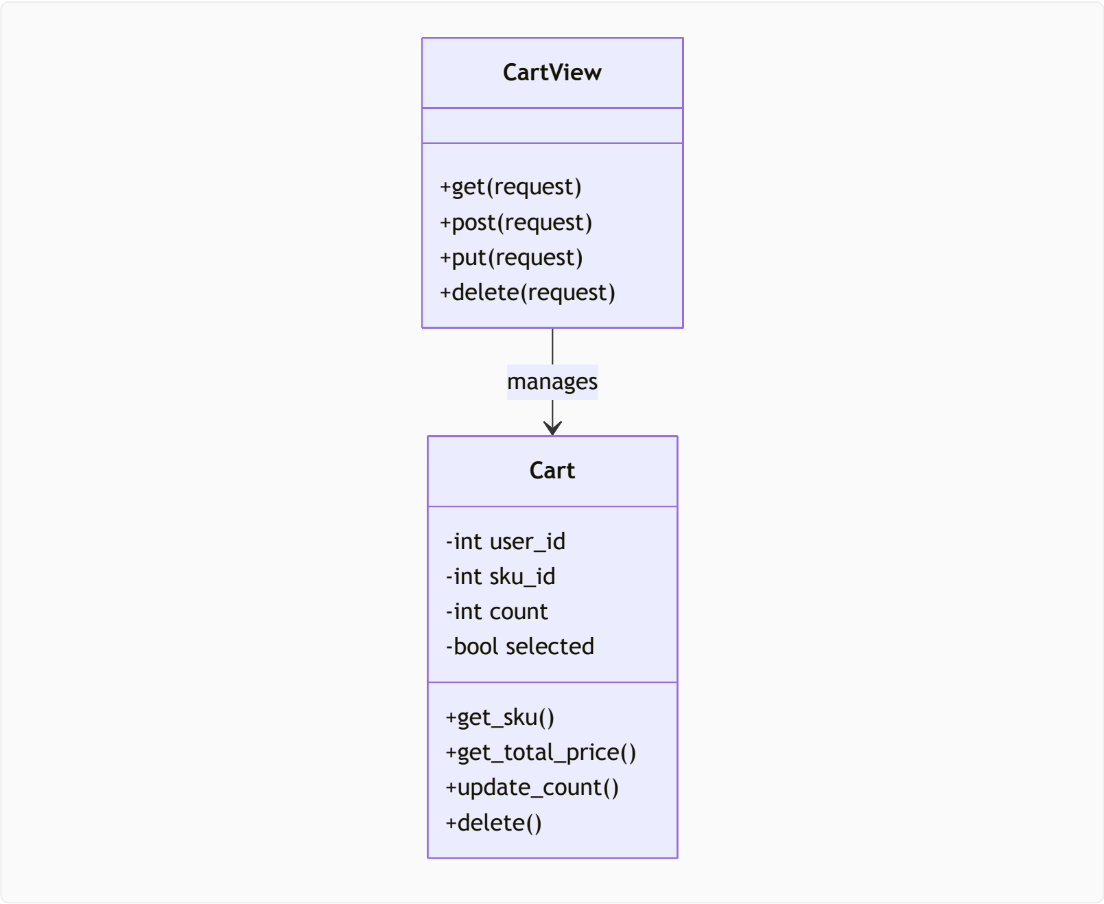
3.5.4 购物车模块内部交互拓扑图
