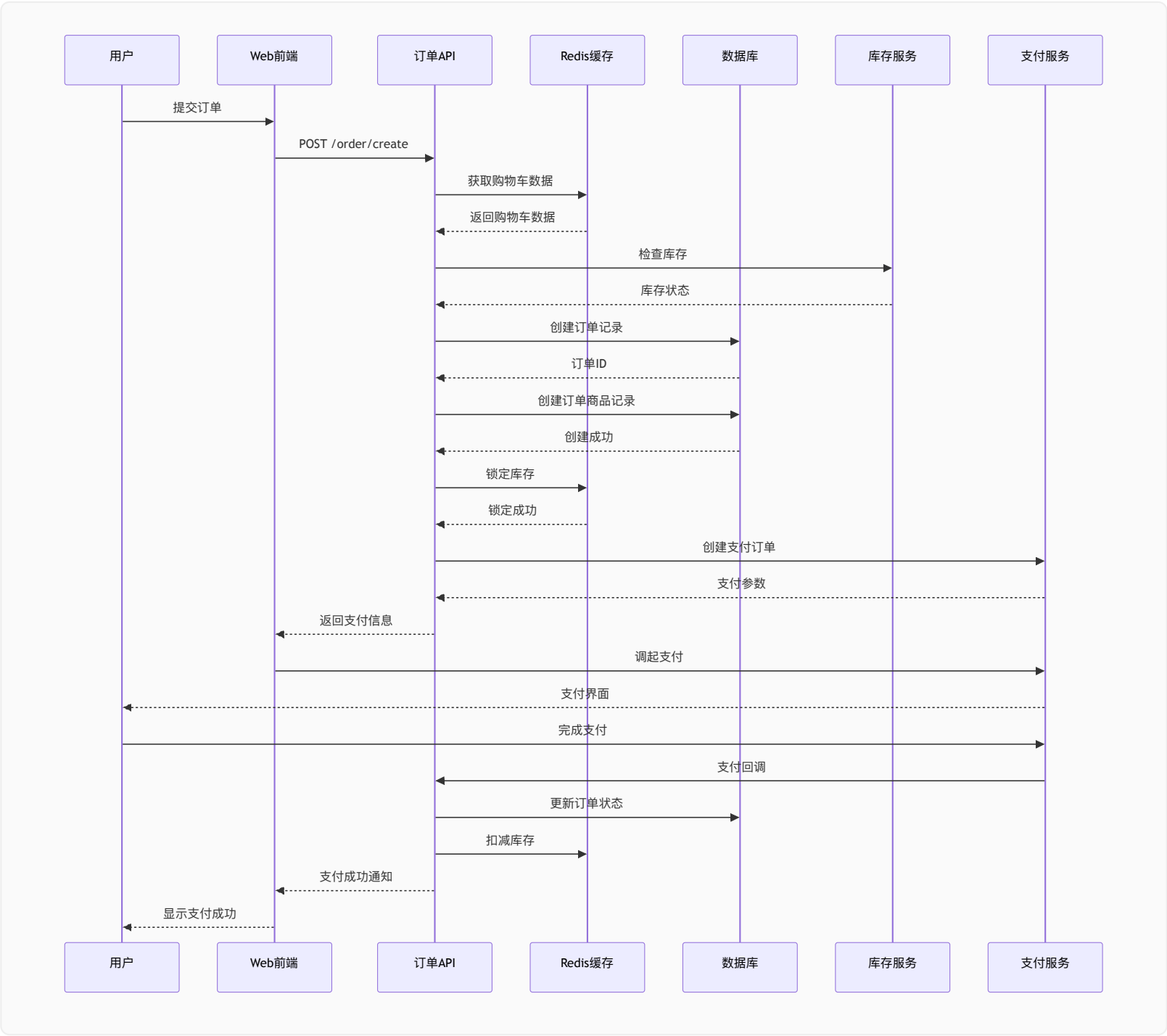
6.5 支付宝支付时序图
