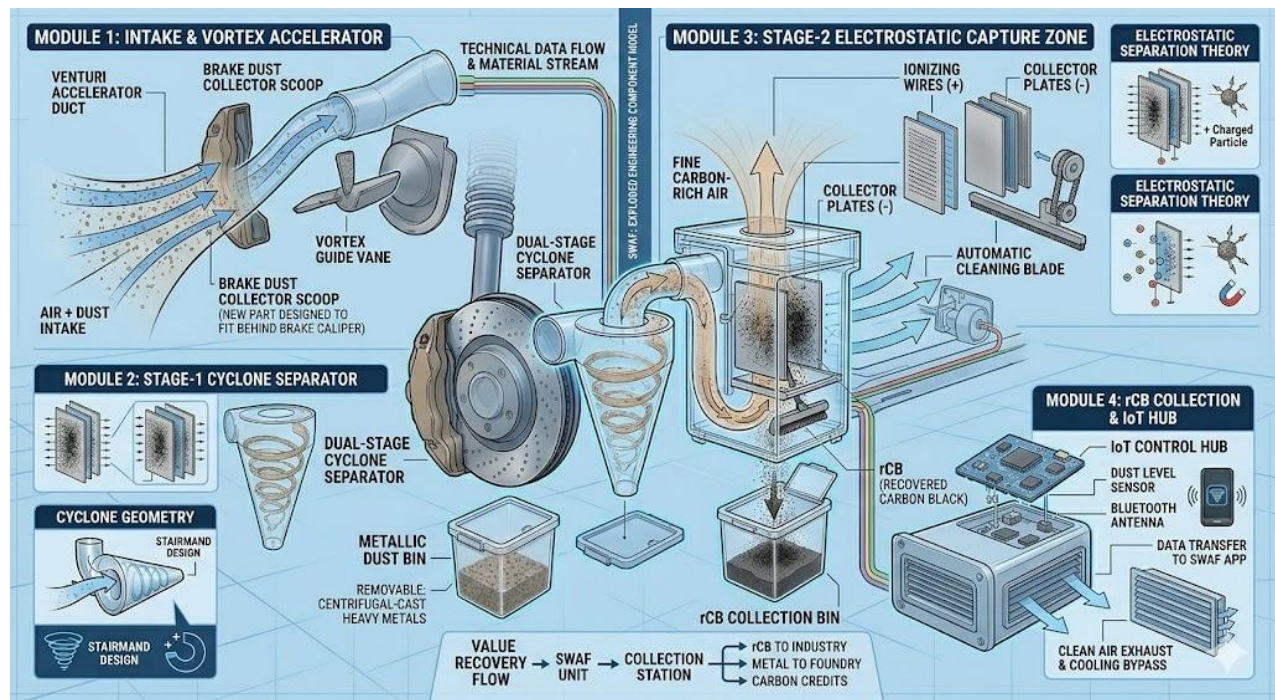
ภาพที่ 5 ต้นแบบเวอร์ชันร่าง
