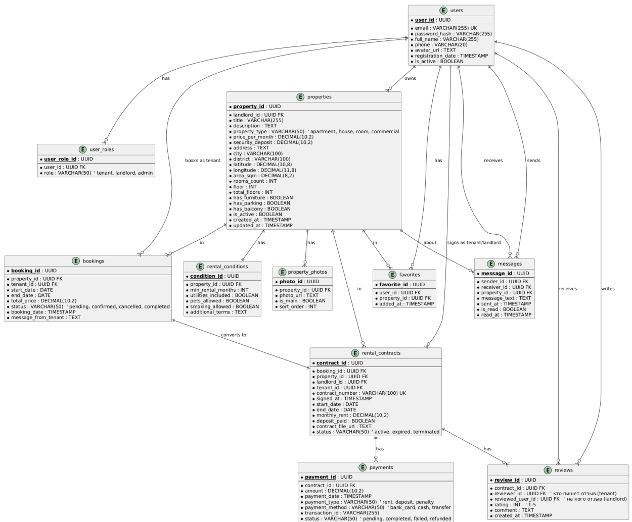
Рисунок 1 — ER-диаграмма базы данных
