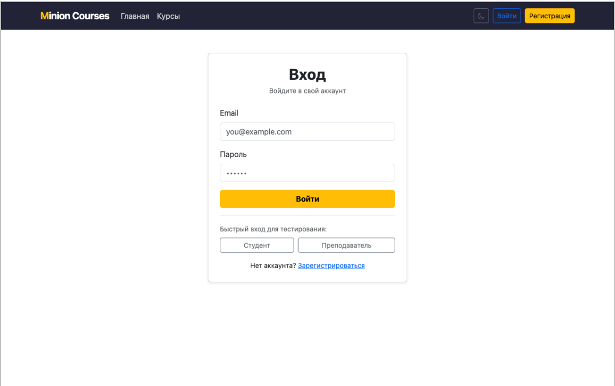
Рис. 2 — Страница входа
