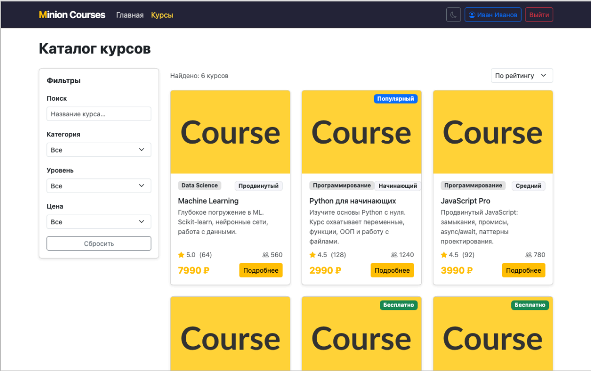
Рис. 5 — Каталог курсов
