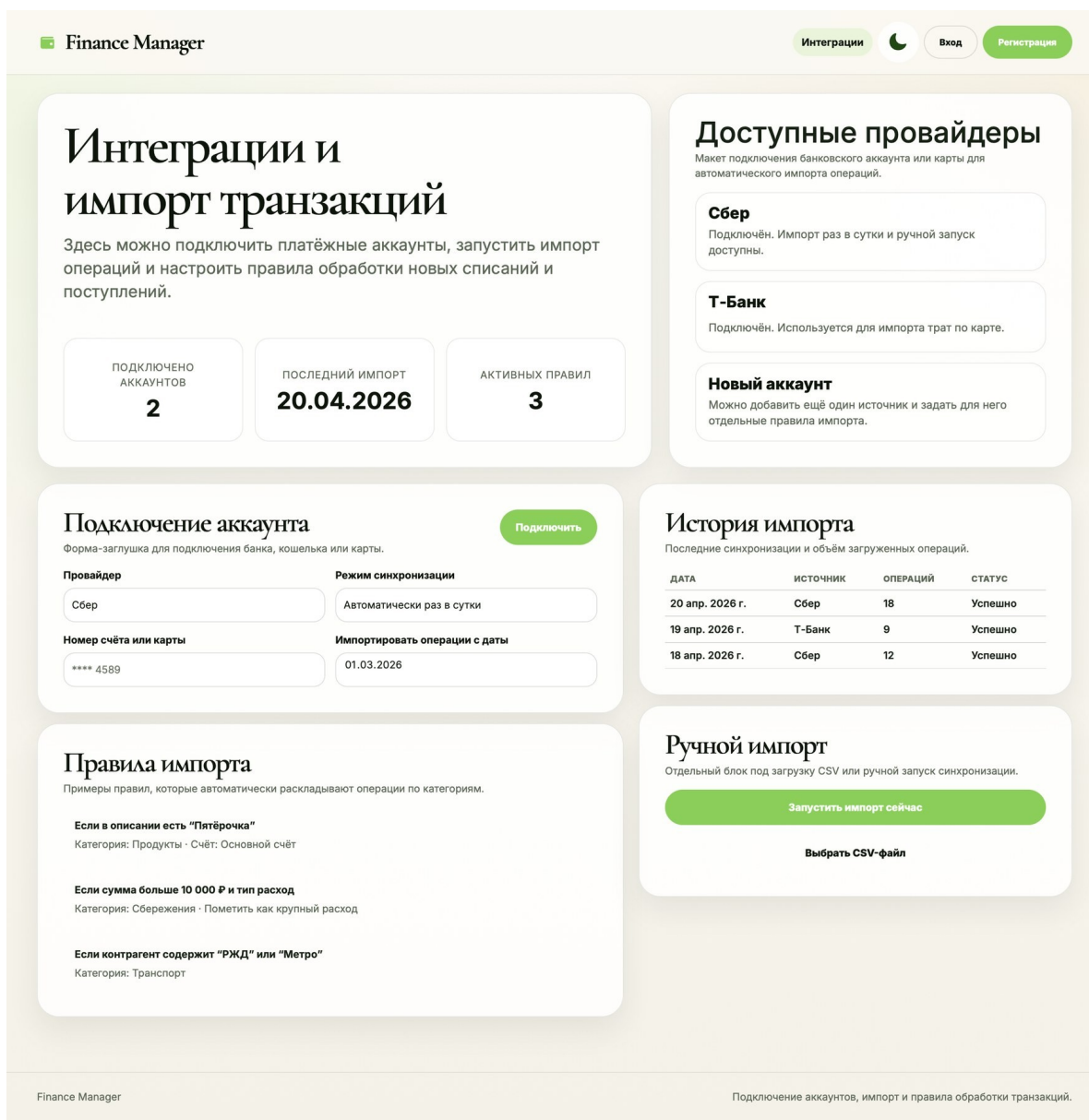
Рисунок 4 - Страница интеграций для импорта операций
