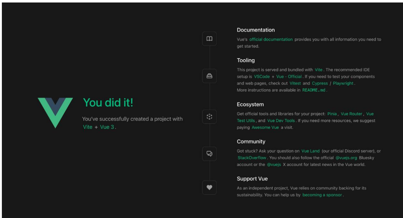
Рис. 2: Запуск приложения
