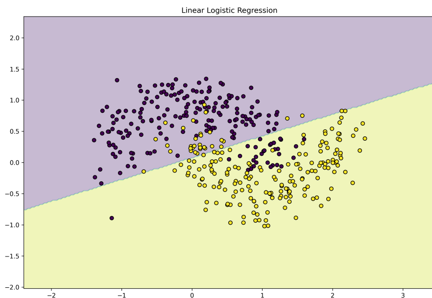
Hình 45: Đường biên quyết định của Logistic Regression cho dữ liệu không phân chia tuyến tính
