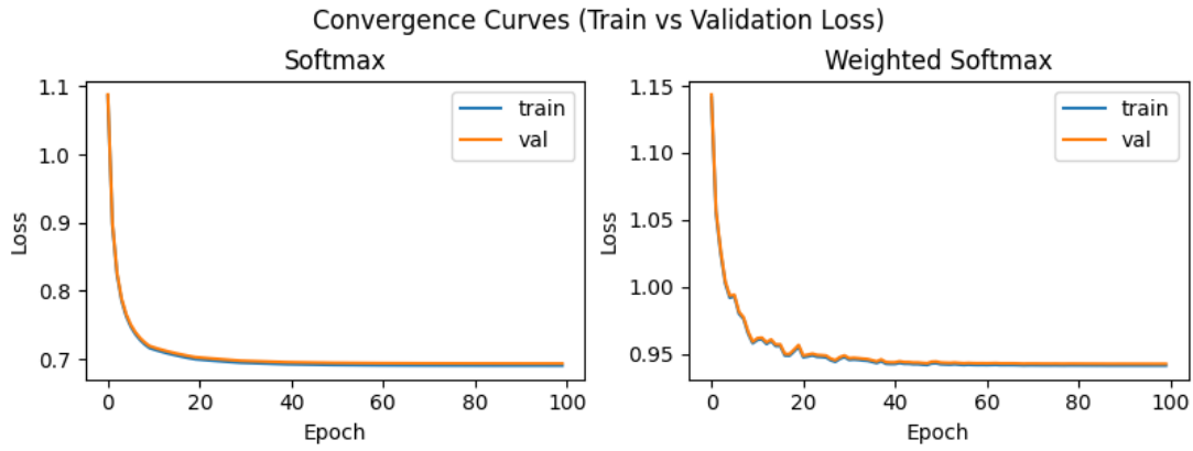
Hình 53: Biểu đồ đường cong lỗi của các mô hình phân lớp sử dụng thuật toán lặp
