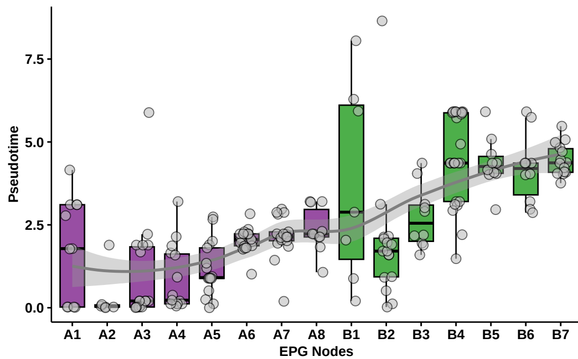
Trajectory: A-B (trend: p=0.00017 )
