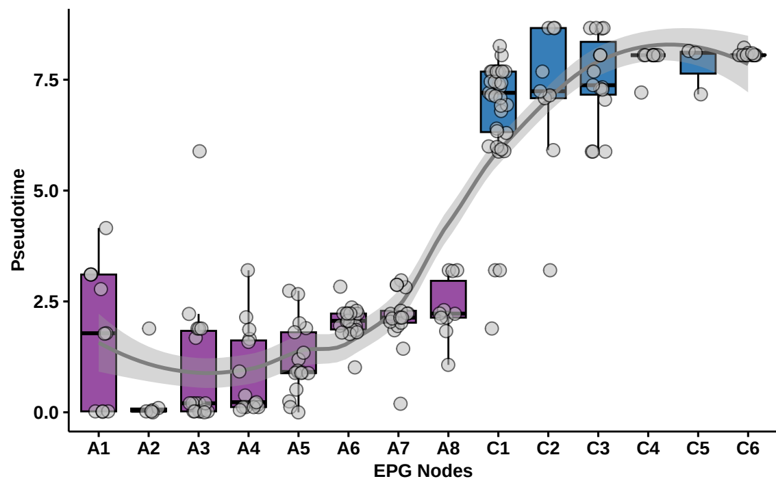
Trajectory: A-C (trend: p=2e-05 )
