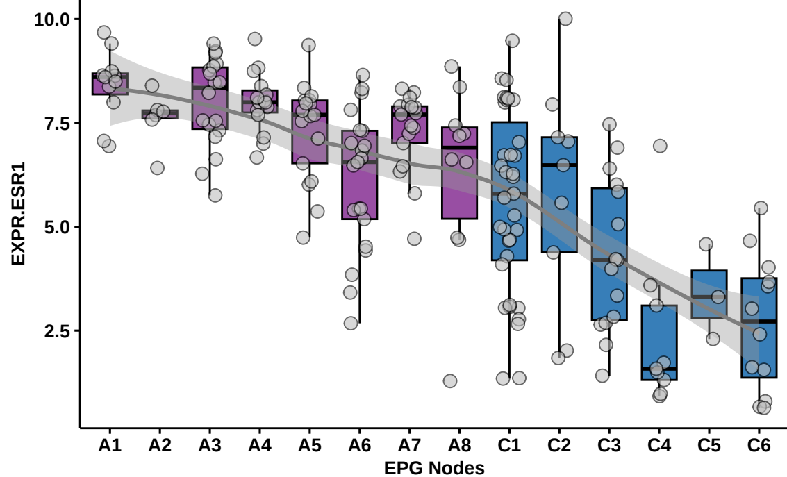
Trajectory: A-C (trend: p=5e-05 )
