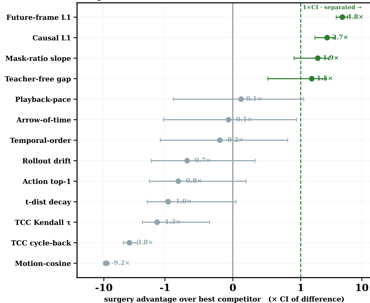
ViT-g · 1B
