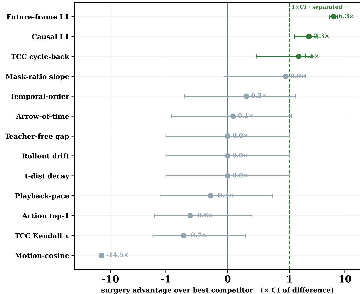
ViT-G · 2B
