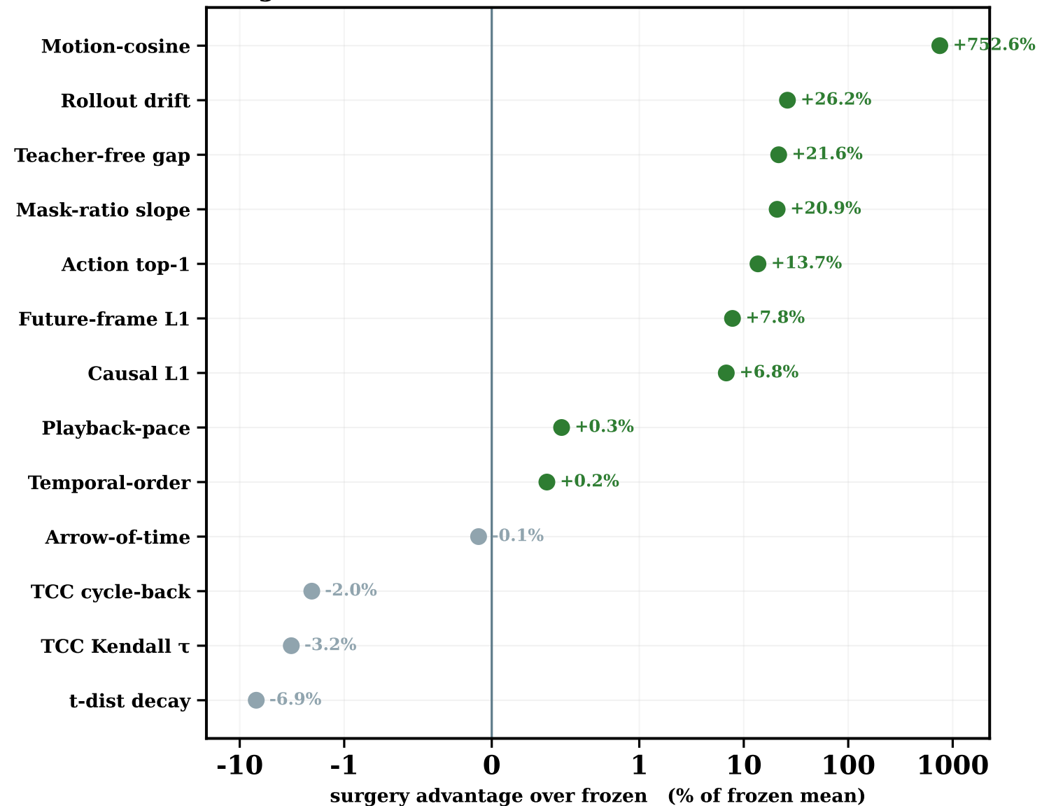
ViT-g · 1B
