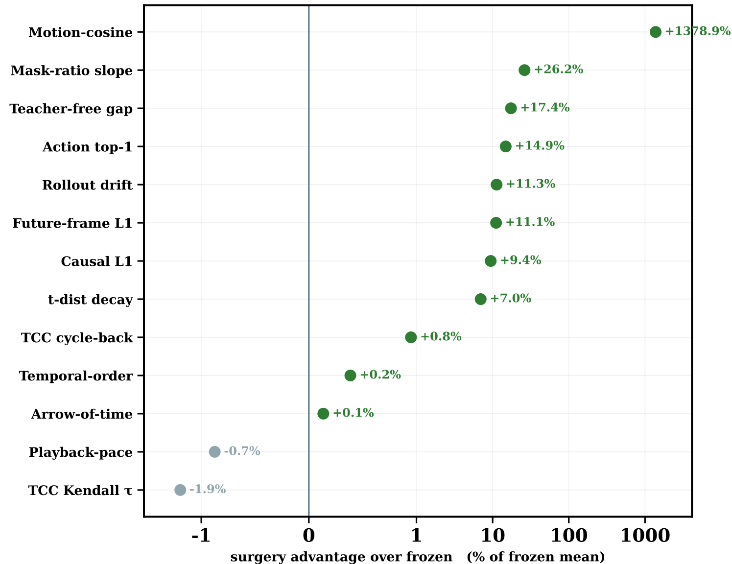
ViT-G · 2B
