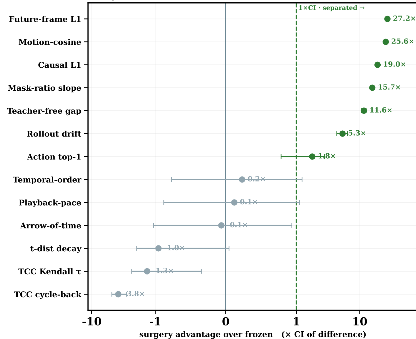
ViT-g · 1B
