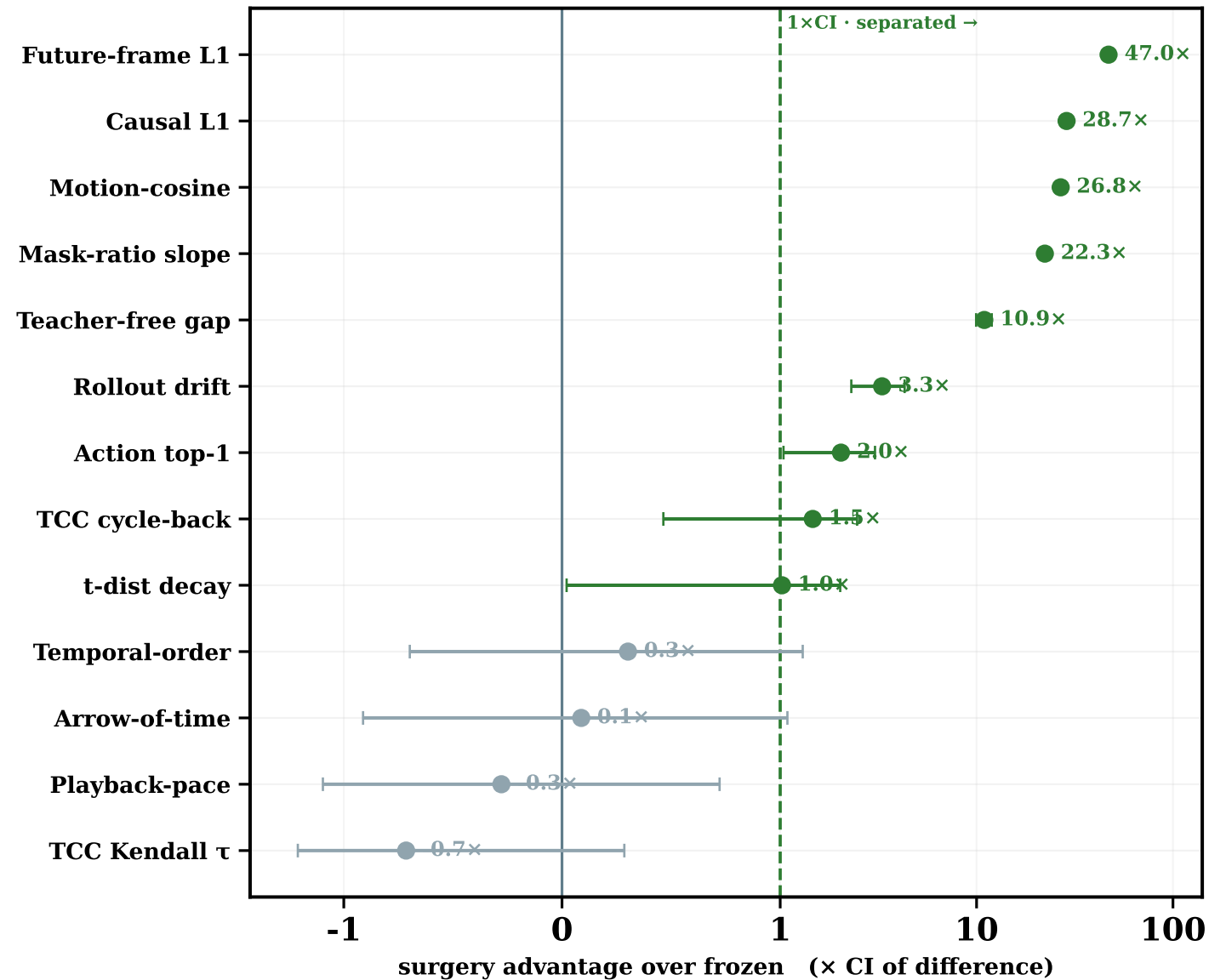
ViT-G · 2B
