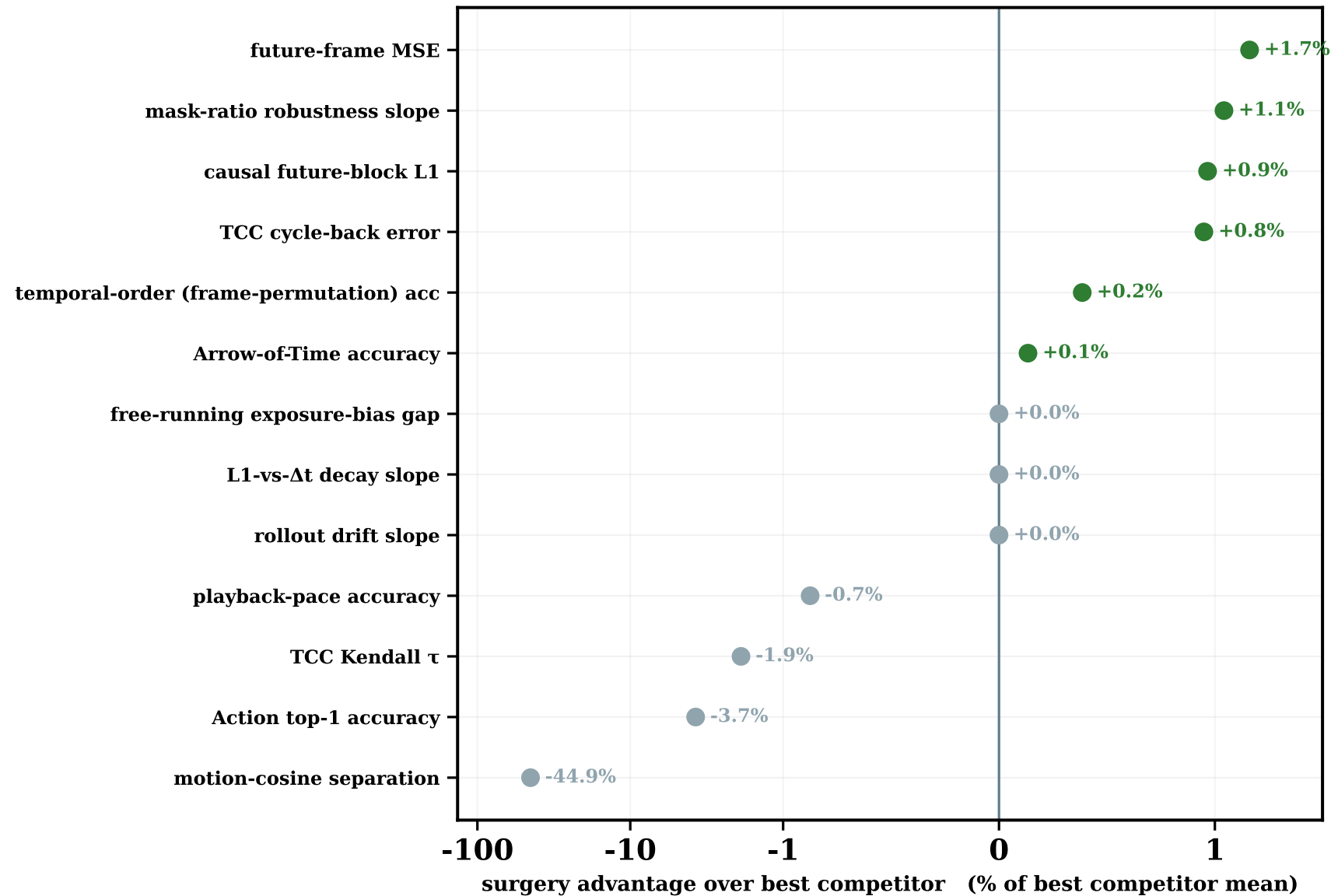
ViT-G · 2B
