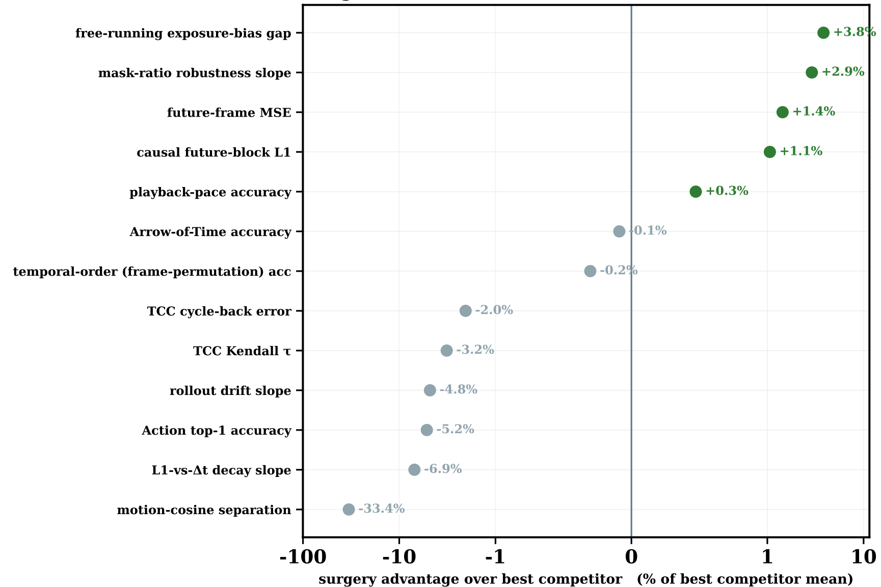
ViT-g · 1B
