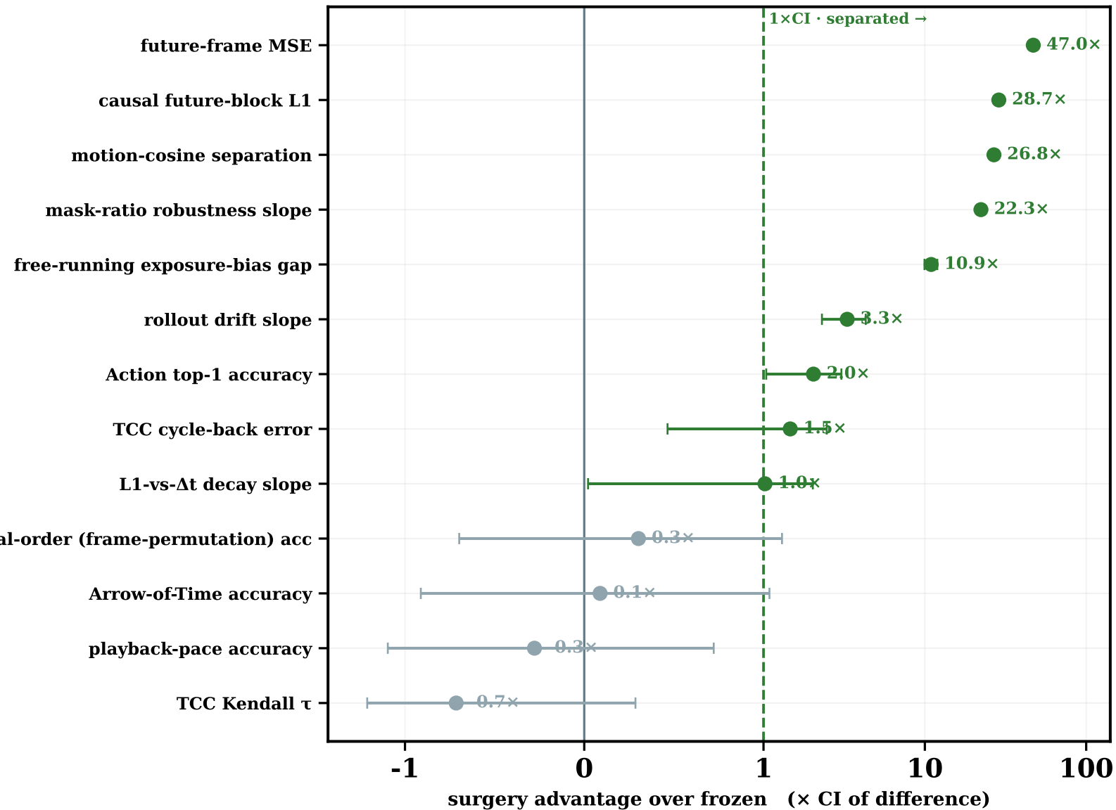
ViT-G · 2B
