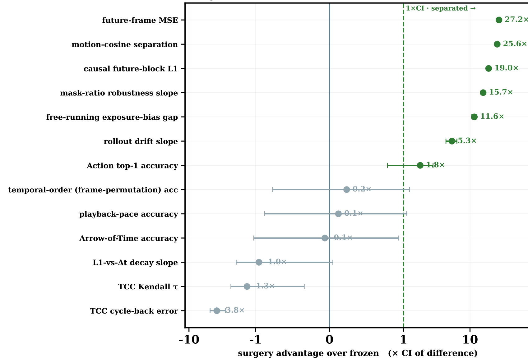
ViT-g · 1B
