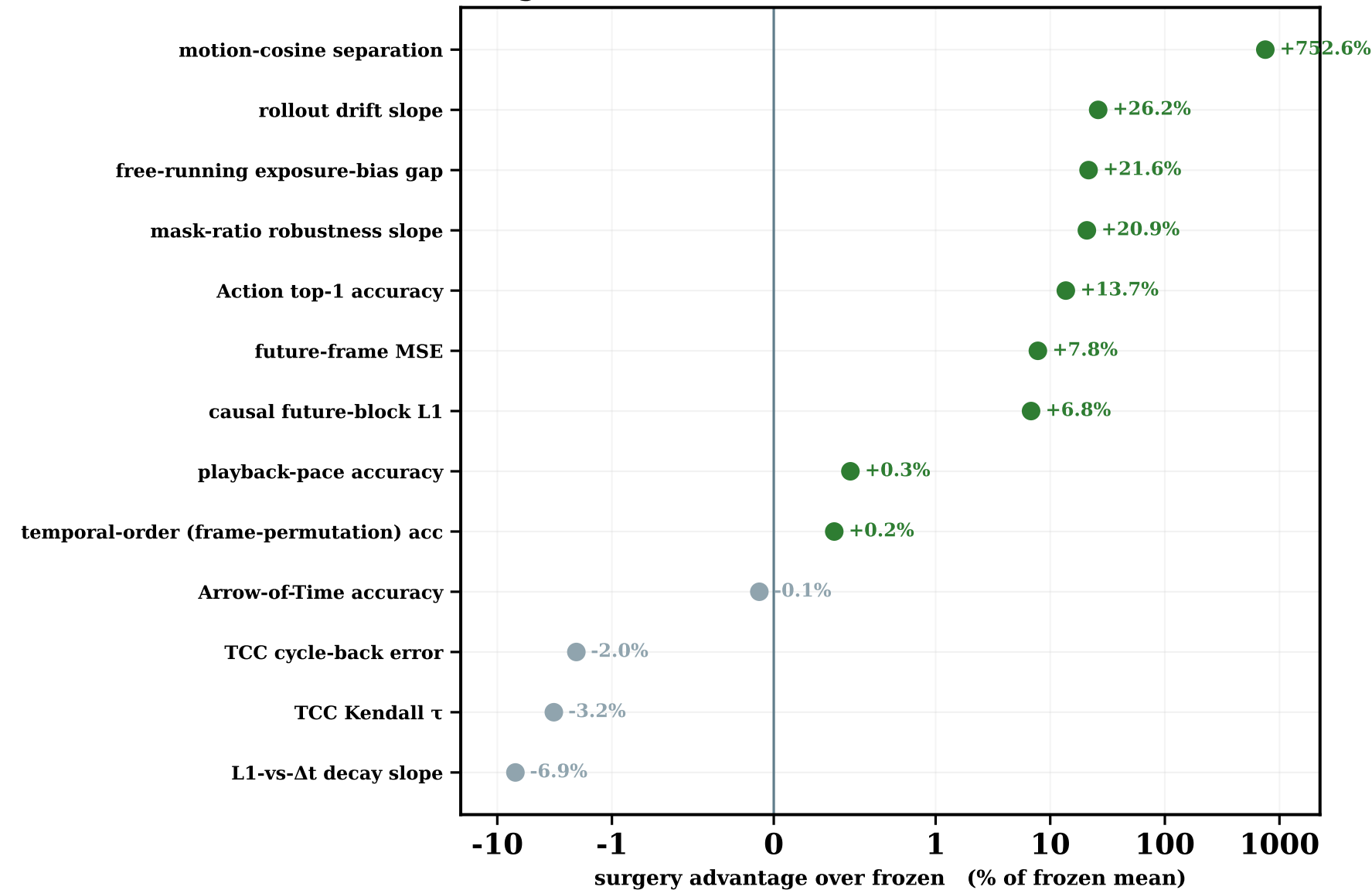
ViT-g · 1B
