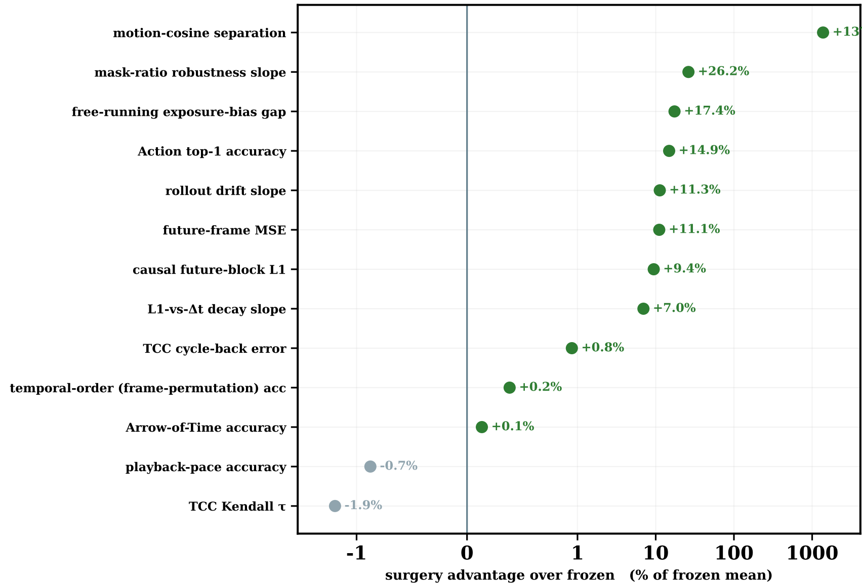
ViT-G · 2B
