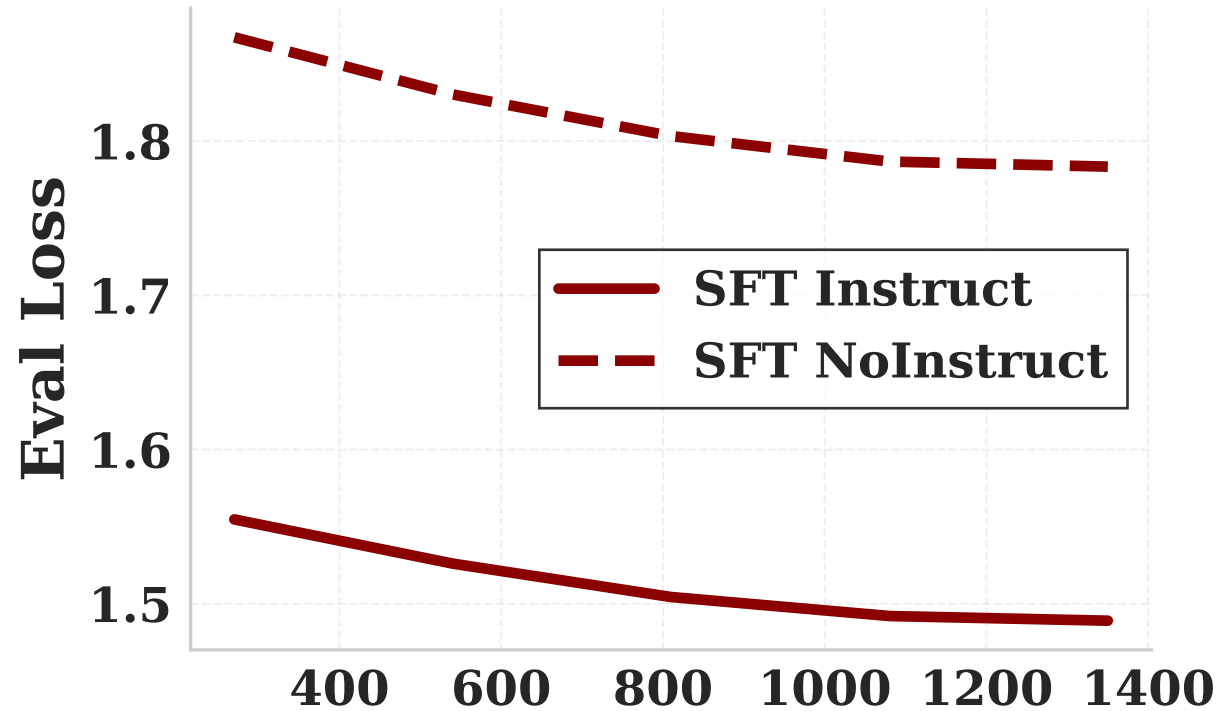
SFT
