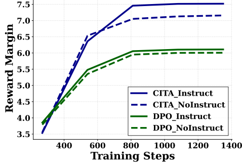
DPO vs CITA: Reward Margins (Llama-3.1-8B)
