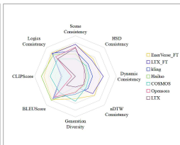
EWMBench arXiv:2505.09694
