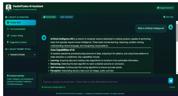
2. Factual Q&A;
