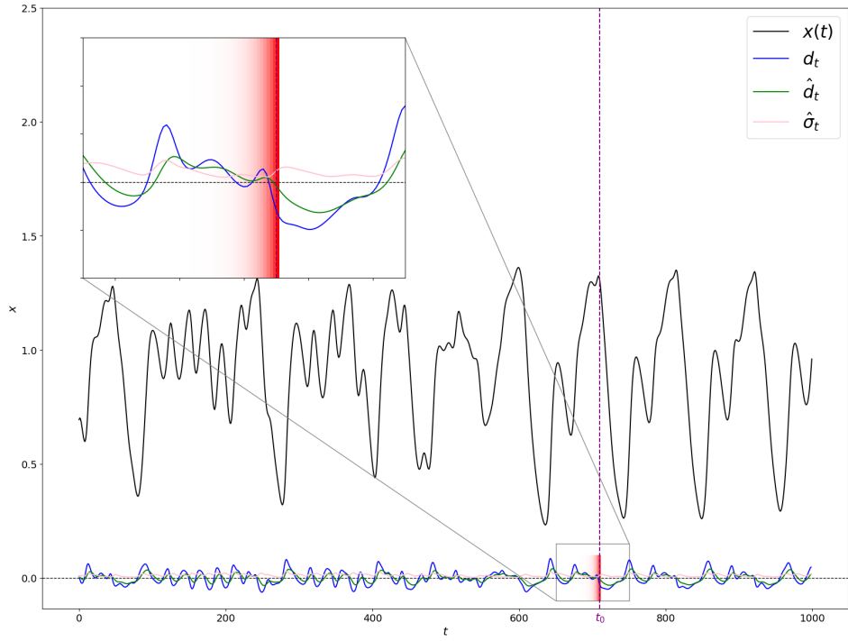
Рисунок 4.7 — График сгенерированной последовательности Mackey-Glass x(t) , t \in [0; 999] с параметрами \tau = 30 , \beta = 0.2 , \gamma = 0.1 , график разностей соседних точек d_t последовательности x(t) , график \hat{d}_t с наложением экспоненциально взвешенного сглаживания на последовательность разностей и график экспоненциально взвешенного скользящего среднеквадратичного отклонения разностей \hat{\sigma}_t . На вложенном изображении участка t \in [650, 750] яркостью красного цвета показано значения весового коэффициента \alpha(1 - \alpha)^{t-p} , p = \overline{1, t_0} из формулы (4.7) при \alpha = 0.2 , определяющего степень вклада предыдущих значений (d_p - \hat{d}_p)^2 в значение \hat{\sigma}_t^2 в точке t . Чем меньше значение \alpha , тем слабее «доверие» к одному лишь значению d_t и тем больше предыдущих значений d_p делают вклад в сглаженное значение
