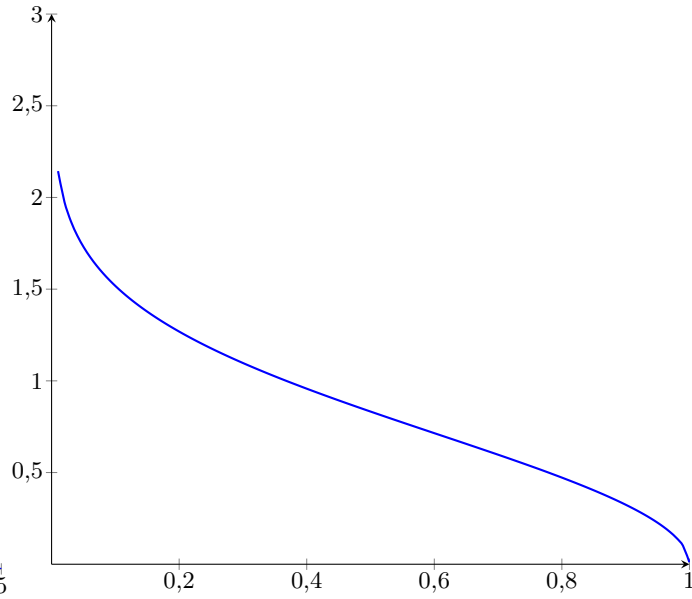
Рисунок 4.4 — График функции \varphi(v) = \sqrt{-\ln v}
