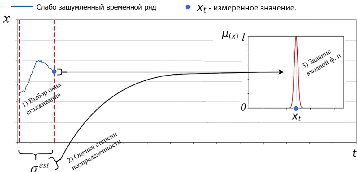
Рисунок 2.7 — Иллюстрация процедуры несинглтонной фаззификации временного ряда с низким уровнем шума
