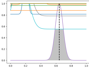
Рисунок 9 — Иллюстрация возникновения «плато» при дефаззификации свертки правил \mu_{B'}(y) (закрашенная область)
