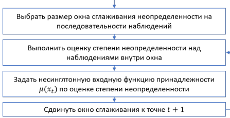
Рисунок 2 — Схема обобщенной процедуры адаптивной несингтонной фаззификации временной последовательности
