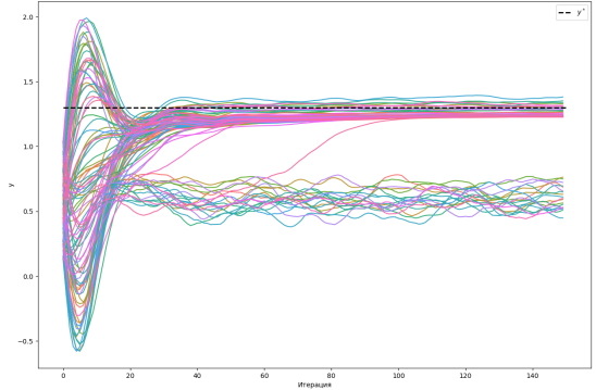
Рисунок 10 — Реализация алгоритма дефаззификации на основе PSO для усреднения по точкам роя, попадающих в плато максимумов
