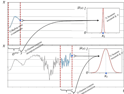
Рисунок 3 — Иллюстрация процедуры несингтонной фаззификации временного ряда с низким (вверху) и высоким (внизу) уровнем шума
