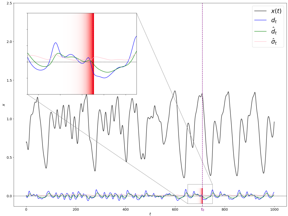
Рисунок 12 — График сгенерированной последовательности Mackey-Glass x(t) , t \in [0; 999] , график разностей соседних точек d_t последовательности x(t) , график \hat{d}_t с наложением экспоненциально взвешенного сглаживания на последовательность разностей и график экспоненциально взвешенного скользящего среднеквадратичного отклонения разностей \hat{\sigma}_t . На вложенном изображении участка t \in [650, 750] яркостью красного цвета показано значения весового коэффициента \alpha(1 - \alpha)^{t-p} , p = \overline{1, t_0} при \alpha = 0.2
