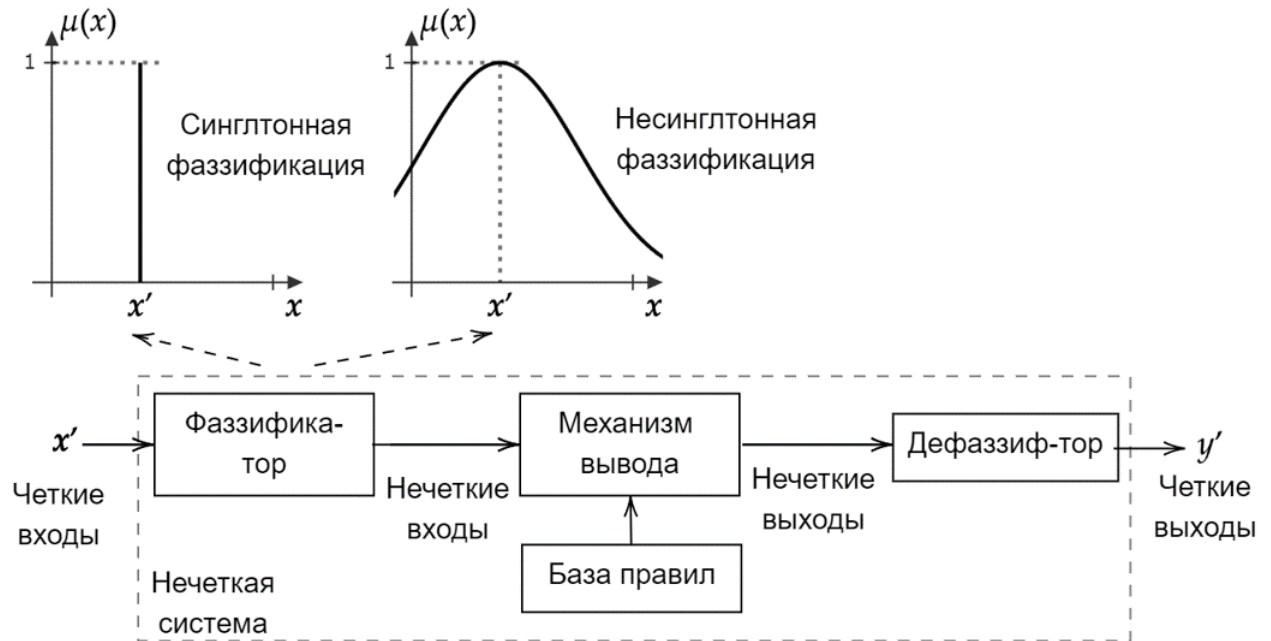
Рисунок 2.1 — Схема системы нечеткого вывода на основе правил с использованием синглотонной и несинглотонной фаззификации
