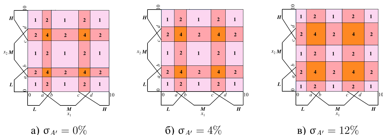
Рисунок 2.2 — Сравнение областей активации правил при переходе от синглотонной фаззификации к несинглотонной и при увеличении ширины области неопределенности \sigma_{A'}
