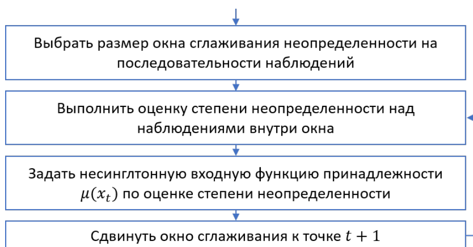
Рисунок 2 — Схема обобщенной процедуры адаптивной несингלטонной фаззификации временной последовательности
